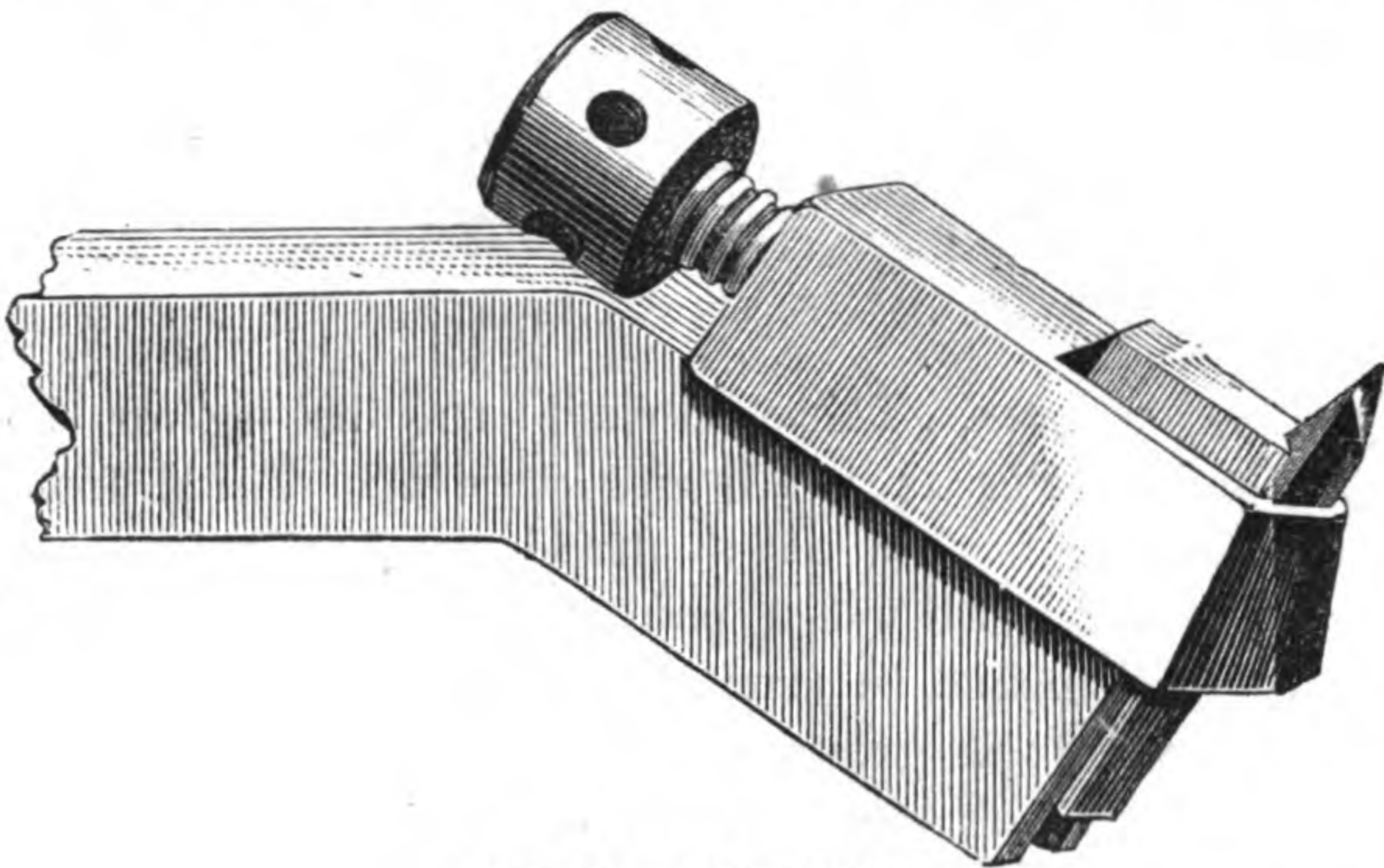
FIG. 18.—HAYDON BAR.
