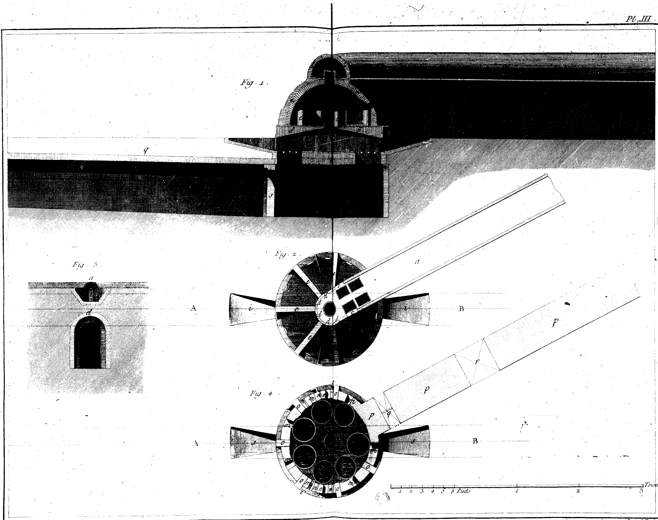
Verrerie en bois, coupe d'un Four de la petite Verrerie à pivotte, sur les lignes A, B, du Plan Géométral; Plans du même Four pris au niveau de l'Arche et 2 au niveau des Pots, et Coupe de la Cave à braise.
