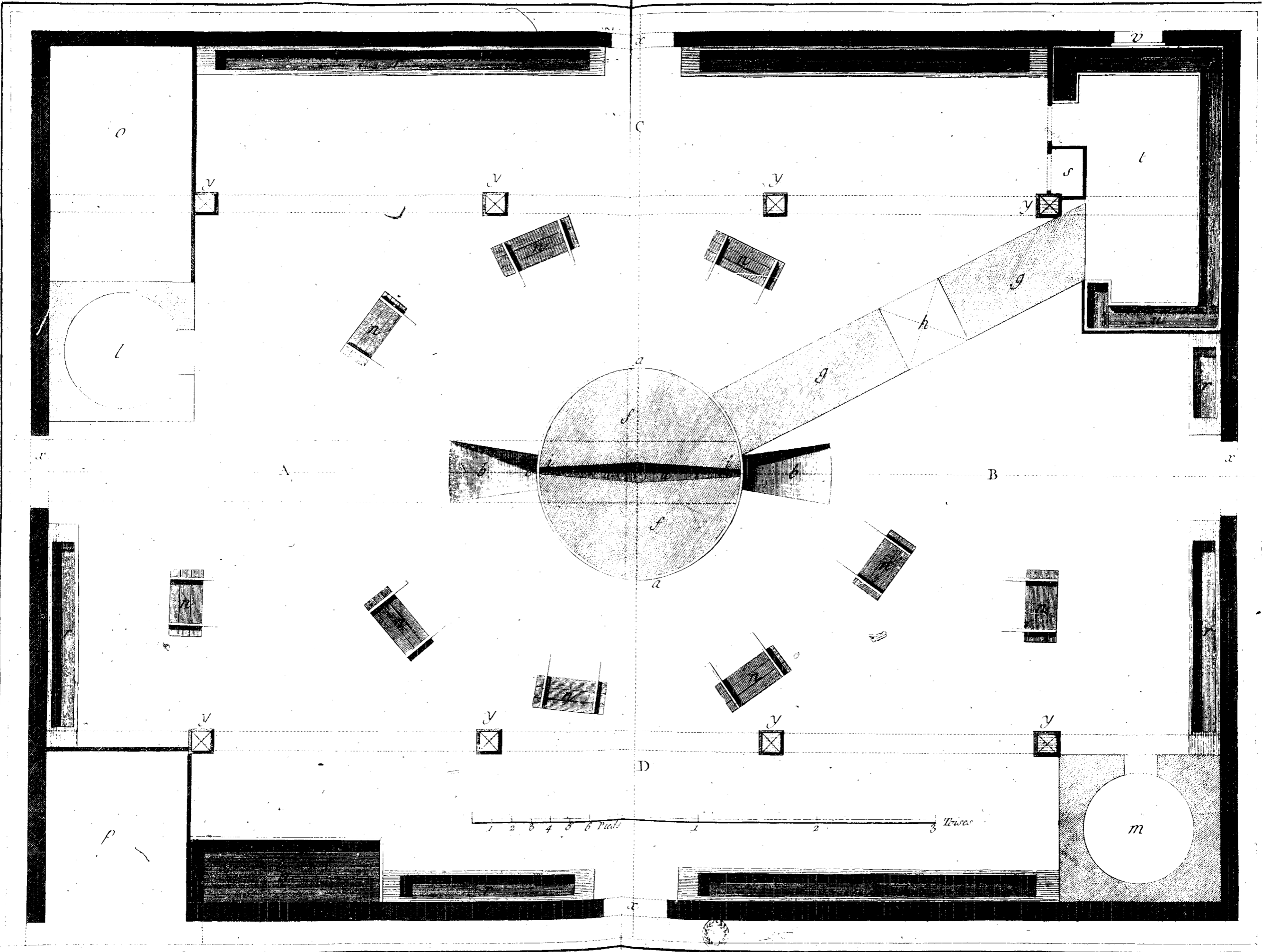
Verrerie en bois, Plan Géométral d'une Halle de petite Verrerie à pivette avec son Four au centre et toutes ses dépendances.
