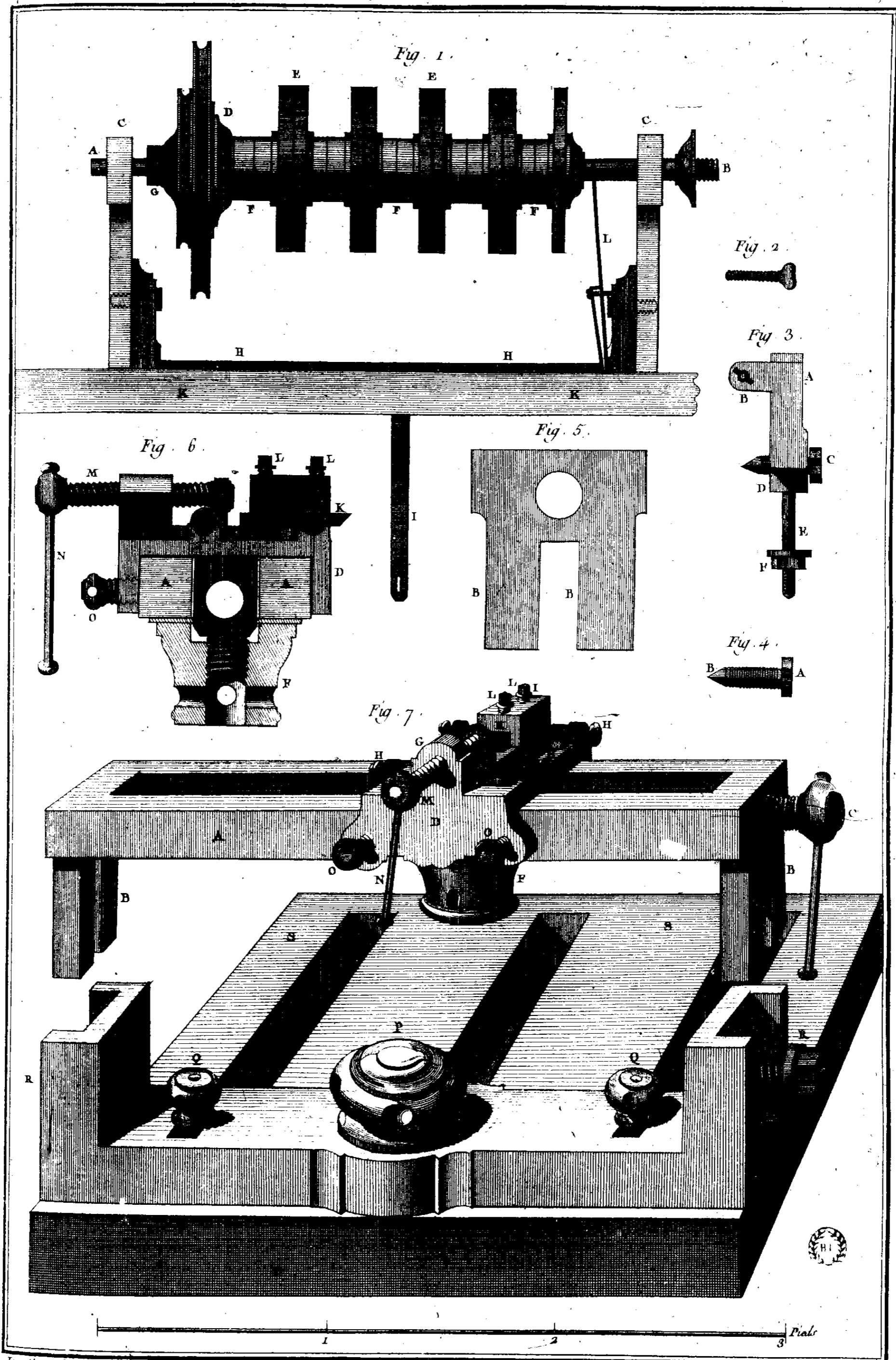
Tourneur, Tour à Guillocher et Supports Composés.
