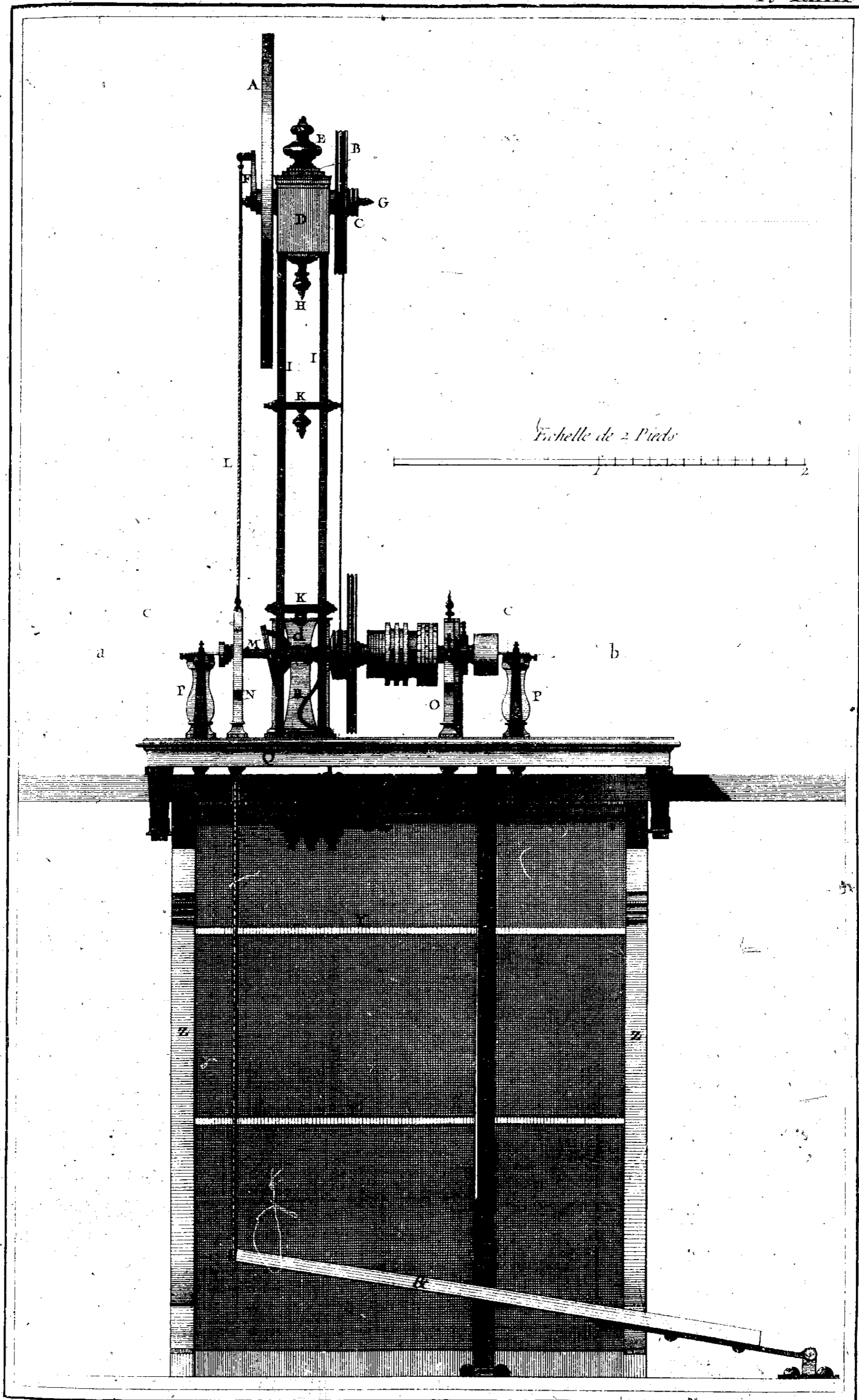
Tourneur, tour à figure, élévation en face
