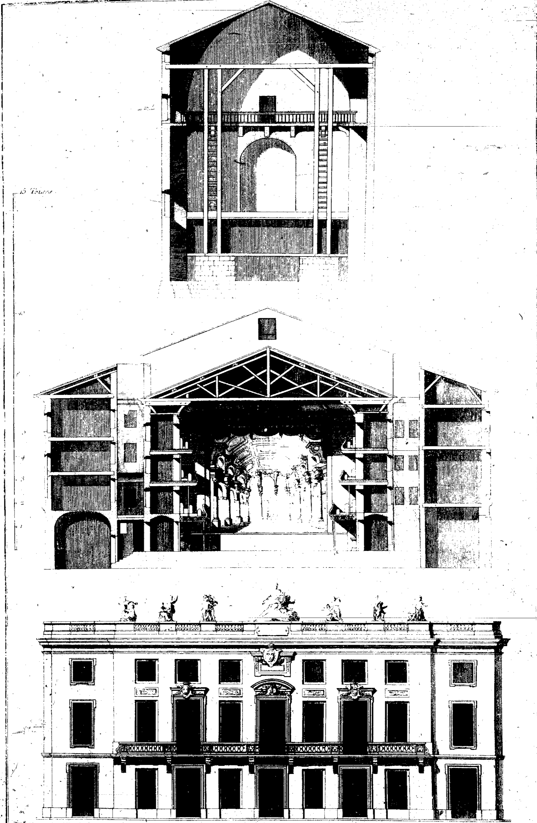
Salles de Spectacles Coupes et Elevations de la Salle de Comedie de Lyon
