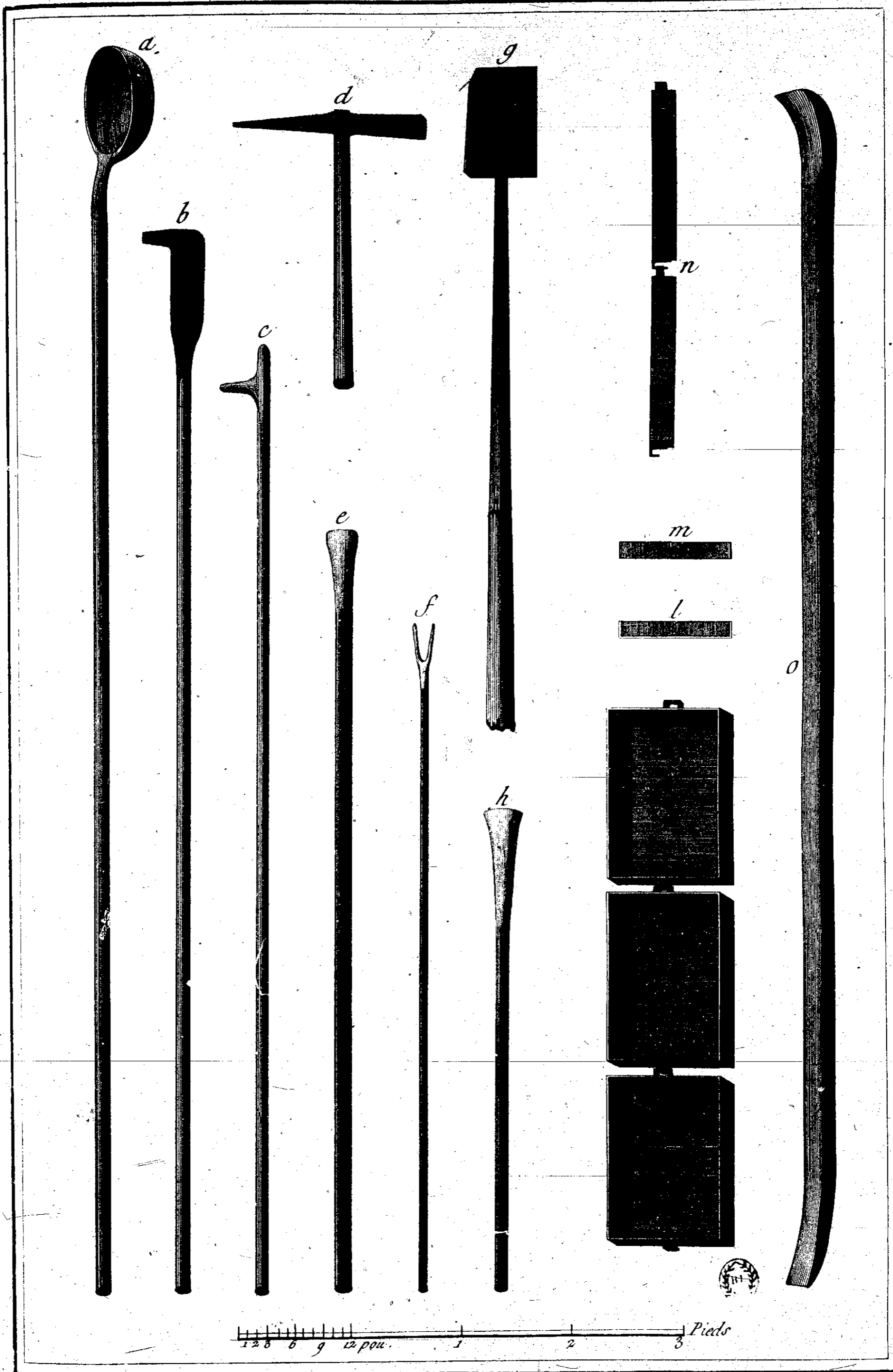
Verrerie en bois, Différens Outils employés dans les petites Verreries à pivotte.
