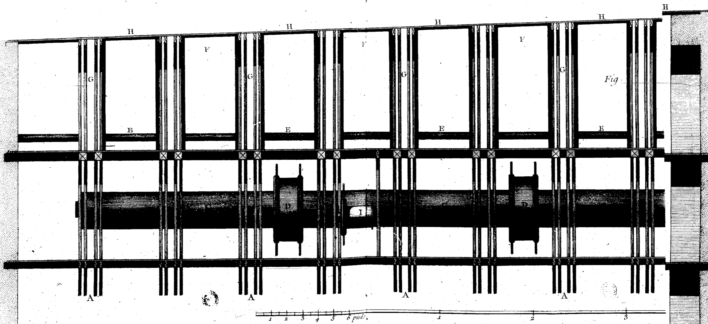
Machines de Théâtres, coupe des deux Planchers du dessous avec la pente du Théâtre.
