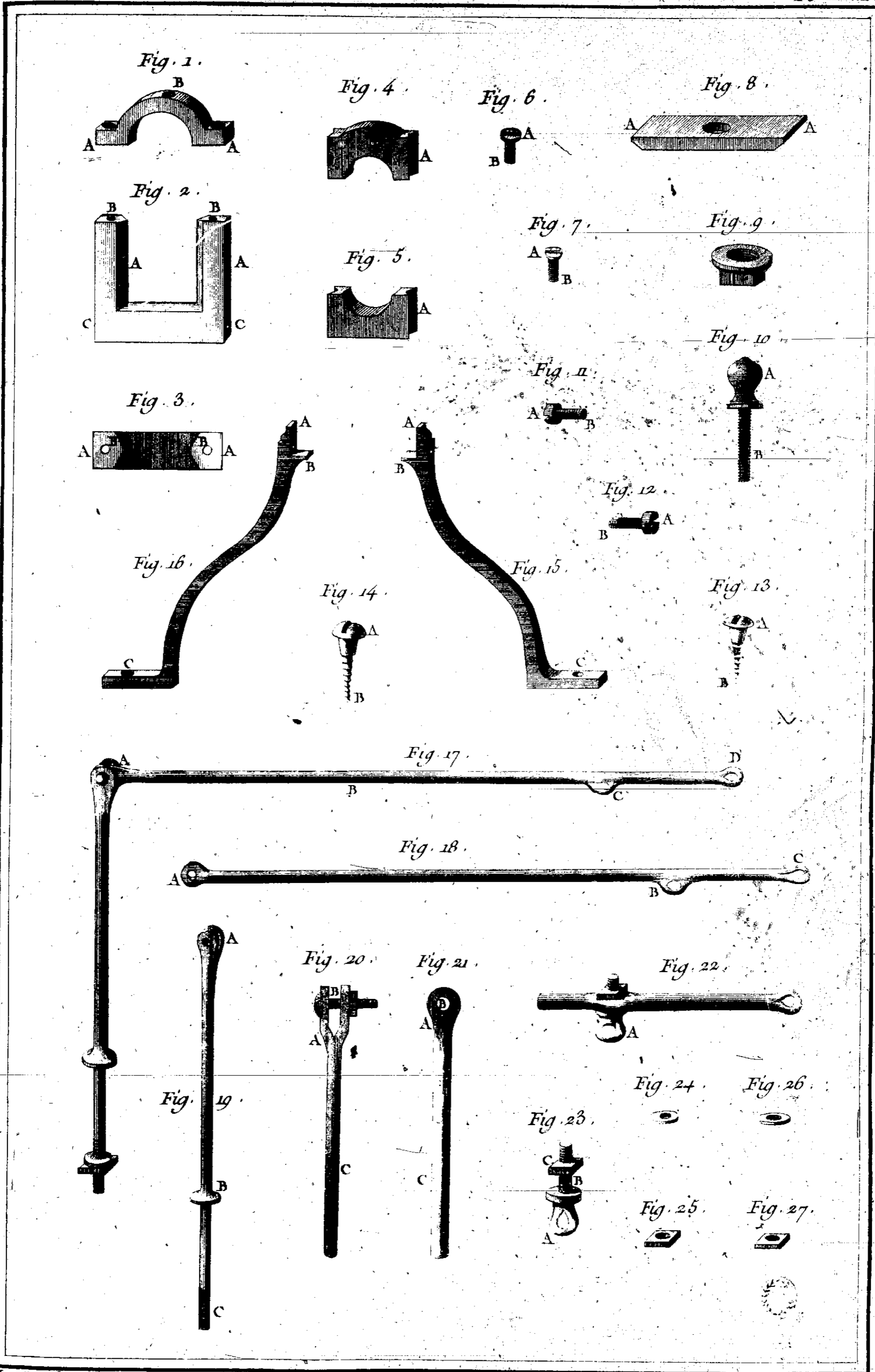
Tourneur, Tour à Figure; Détails de l'un des Supports de renvoi et Bascule de la Pédale.
