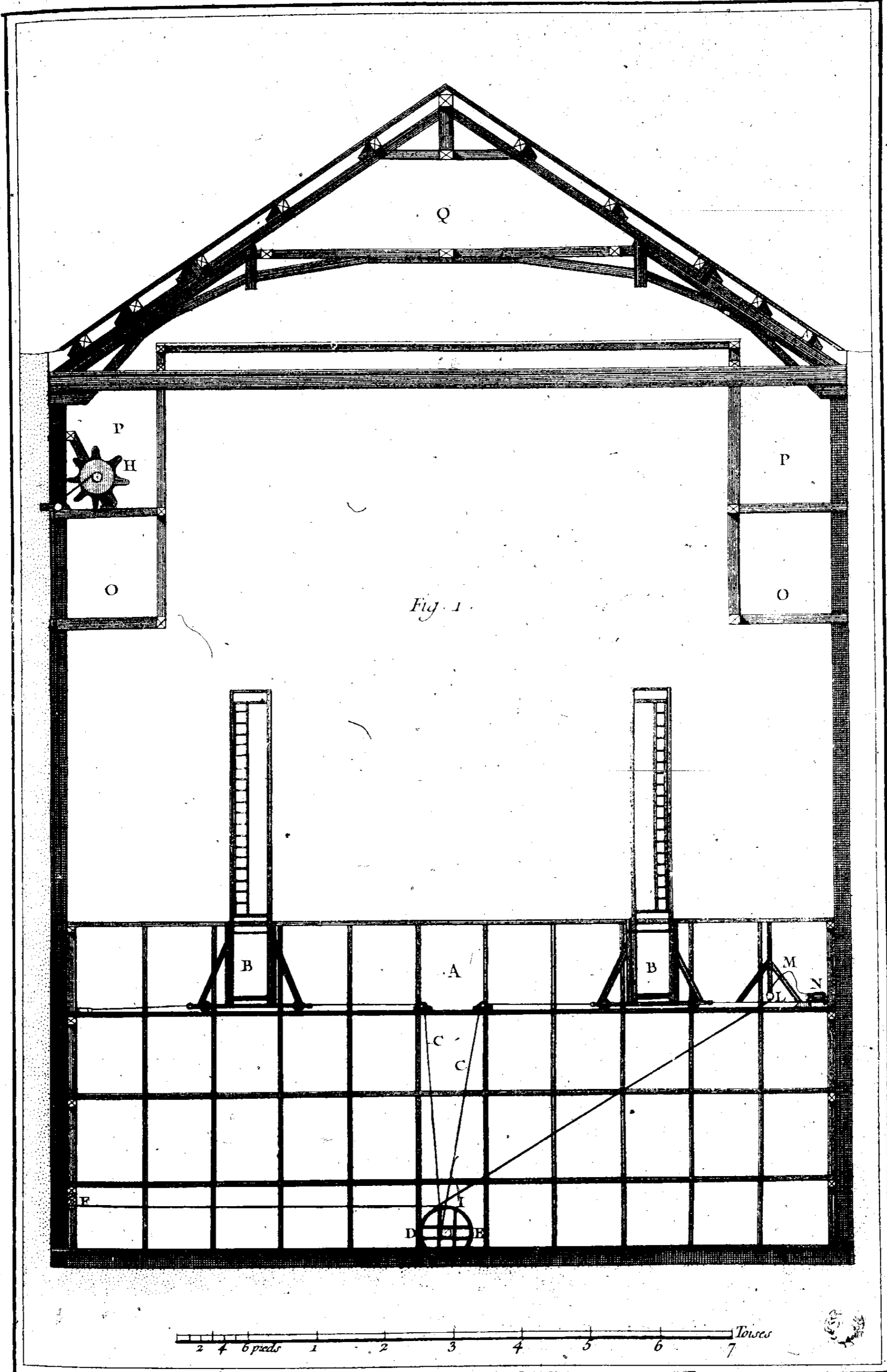
Machines de Théâtres, Coupe sur toute la hauteur et la largeur du Théâtre avec le Développement pour le changement des faux Chassis.
