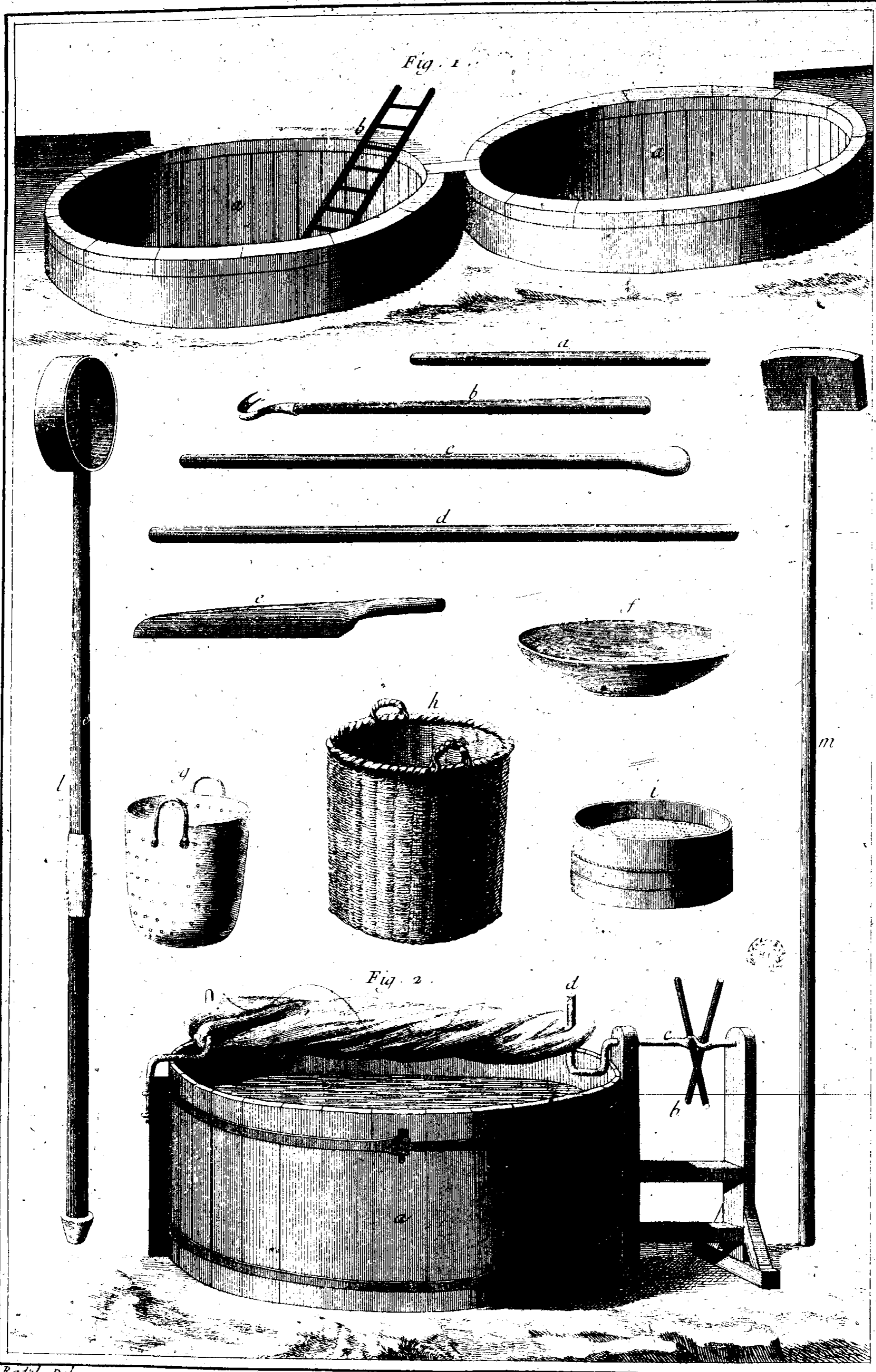
Teinture des Gobelins, Tordoir, Outils et Cuvées.
