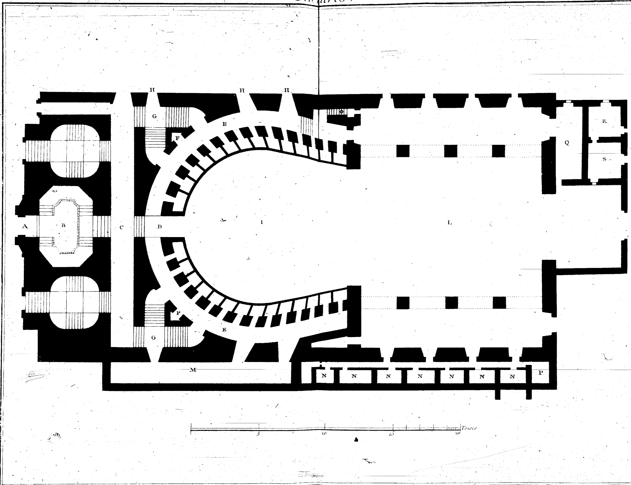
Salles de Spectacles, Plan du Theatre Royal de S t . Charles a Naples
