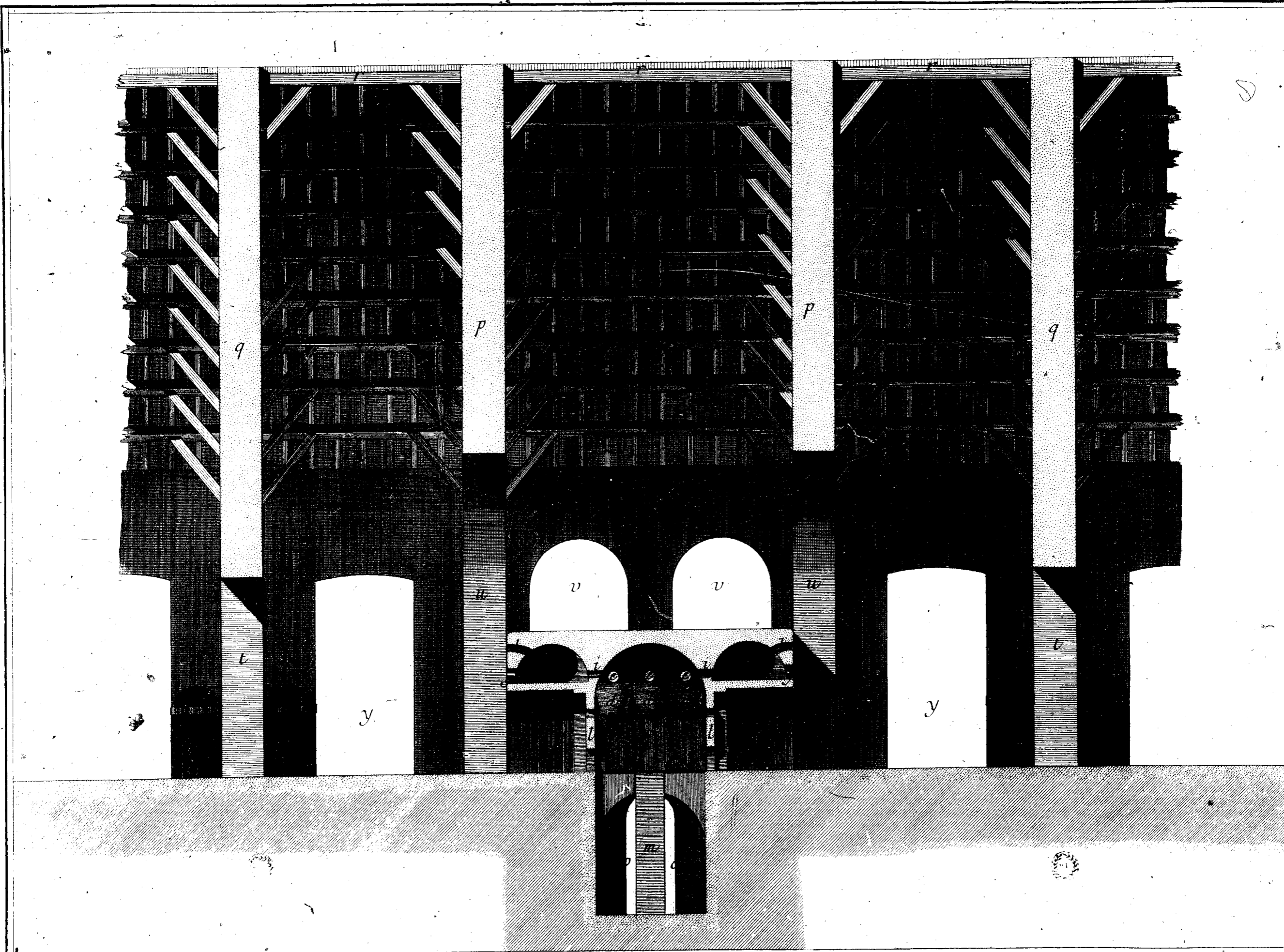
Verrerie en Bouteilles, chauffée en Charbon de Terre. Coupe sur la longueur d'une des quatre Halles et de son Four, de la Verrerie Royale de Seve près Paris.
