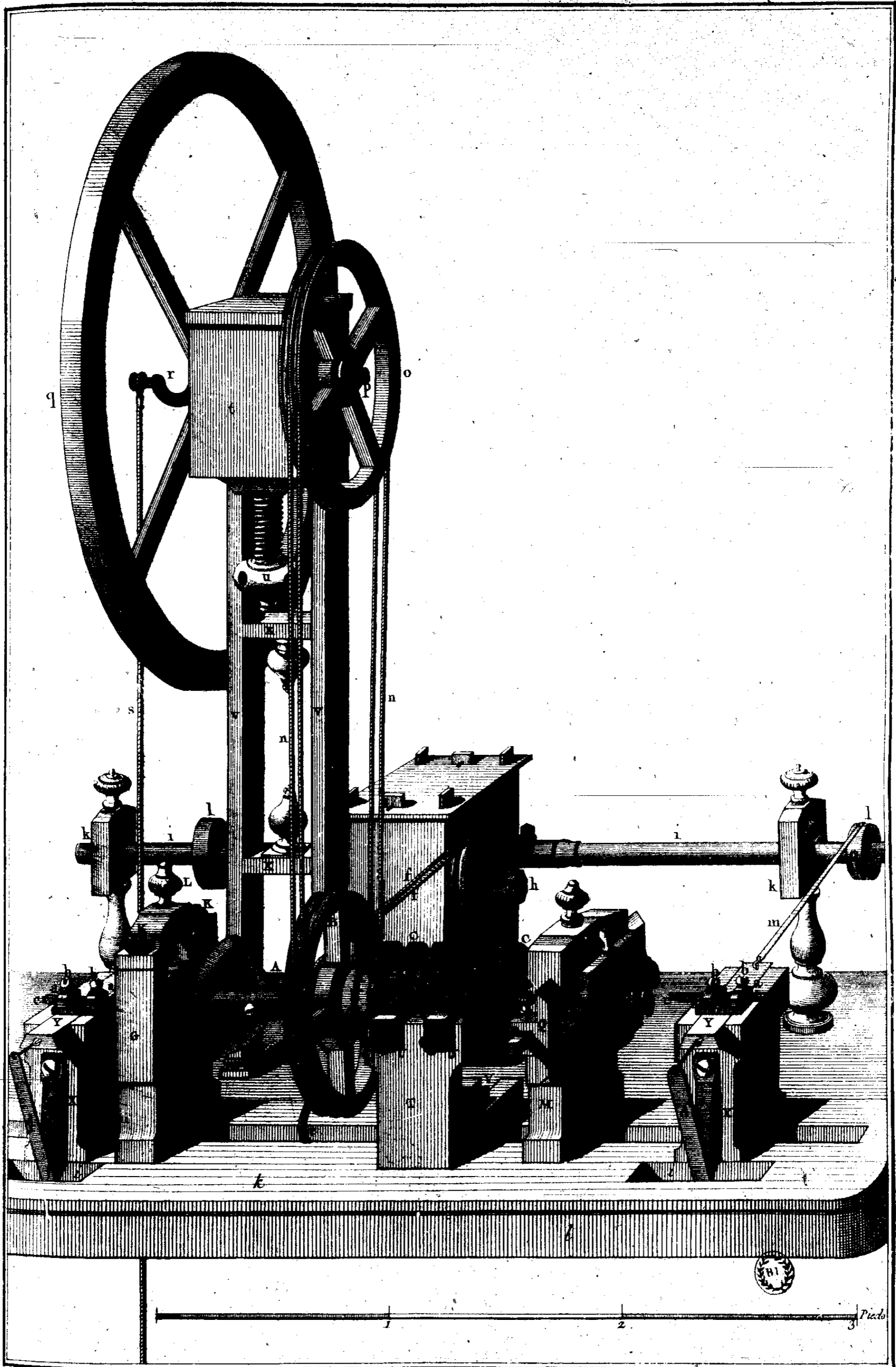
Tourneur, Tour à Roue à Guallochis et Outils mobiles.
