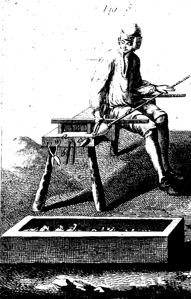
Verrerie en bois, l'opération de remuer la Composition dans le Pot de fonte, de cueillir la matiere ou Poste, de la rouler sur le marbre, de la souffler dans le moule, et autres opérations relatives à la façon d'un verre.
