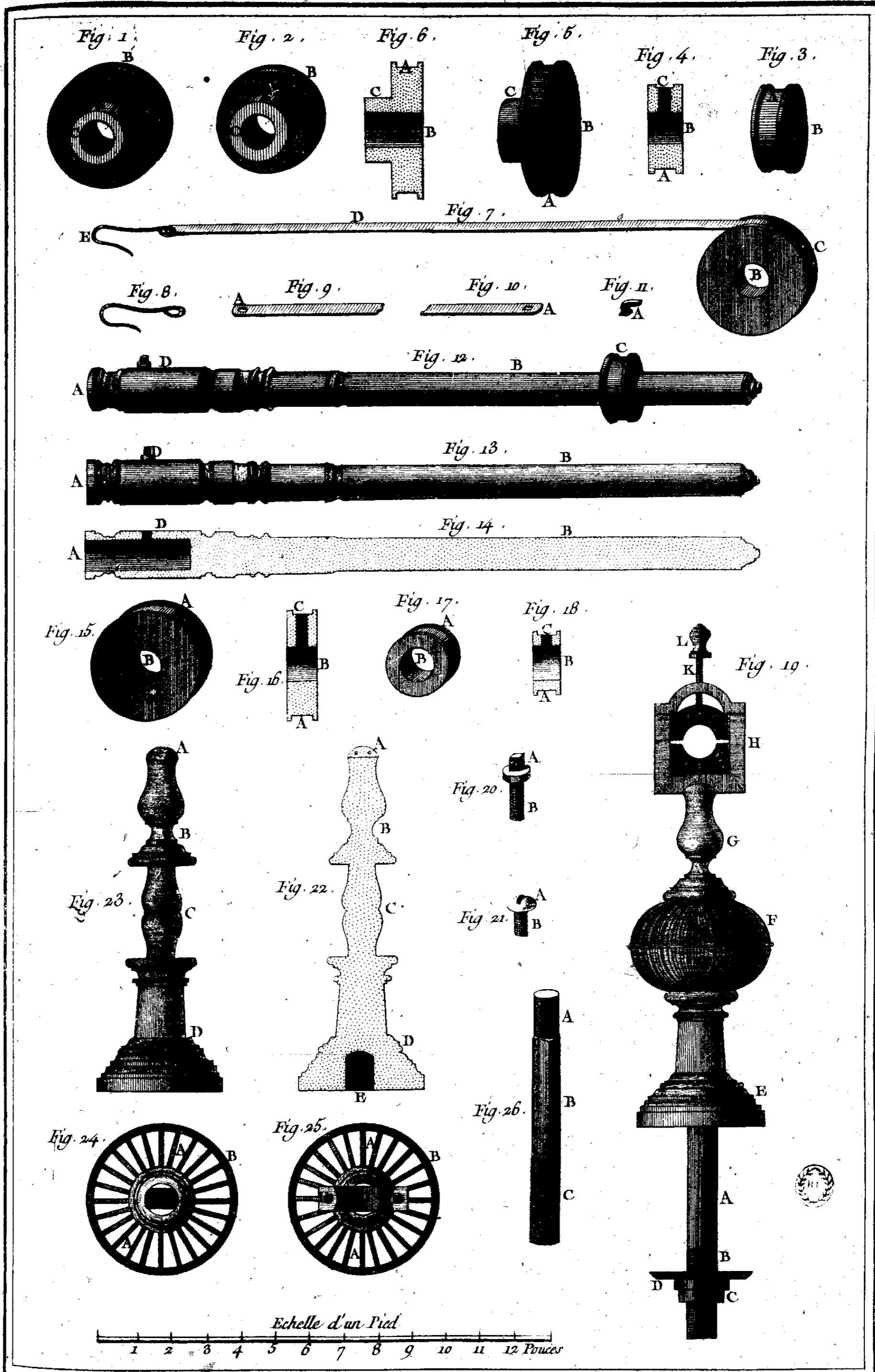
Tourneur, Tour à Figure. Détails de l'Arbre de renvoi et l'un de ses Supports.
