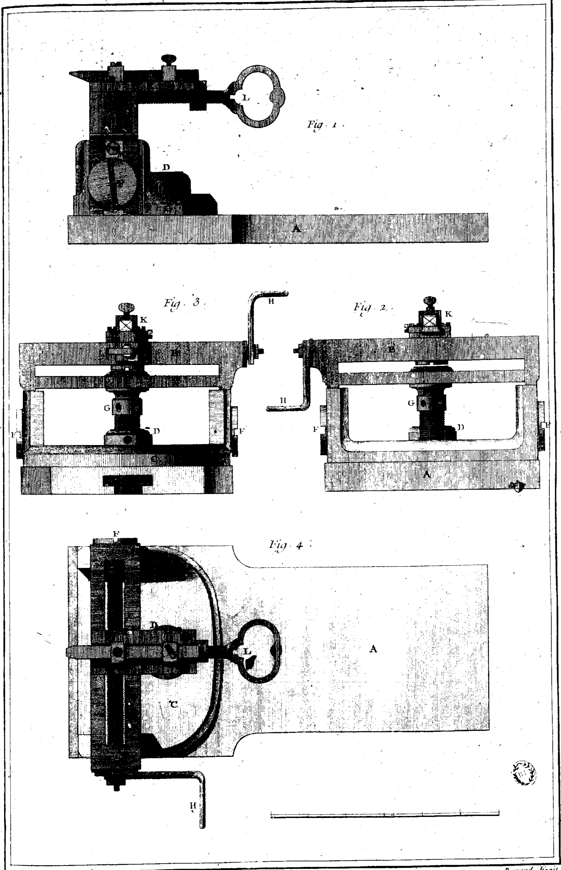
Tourneur, Tour à Figure; Support à pivot portant outil à travailler.
