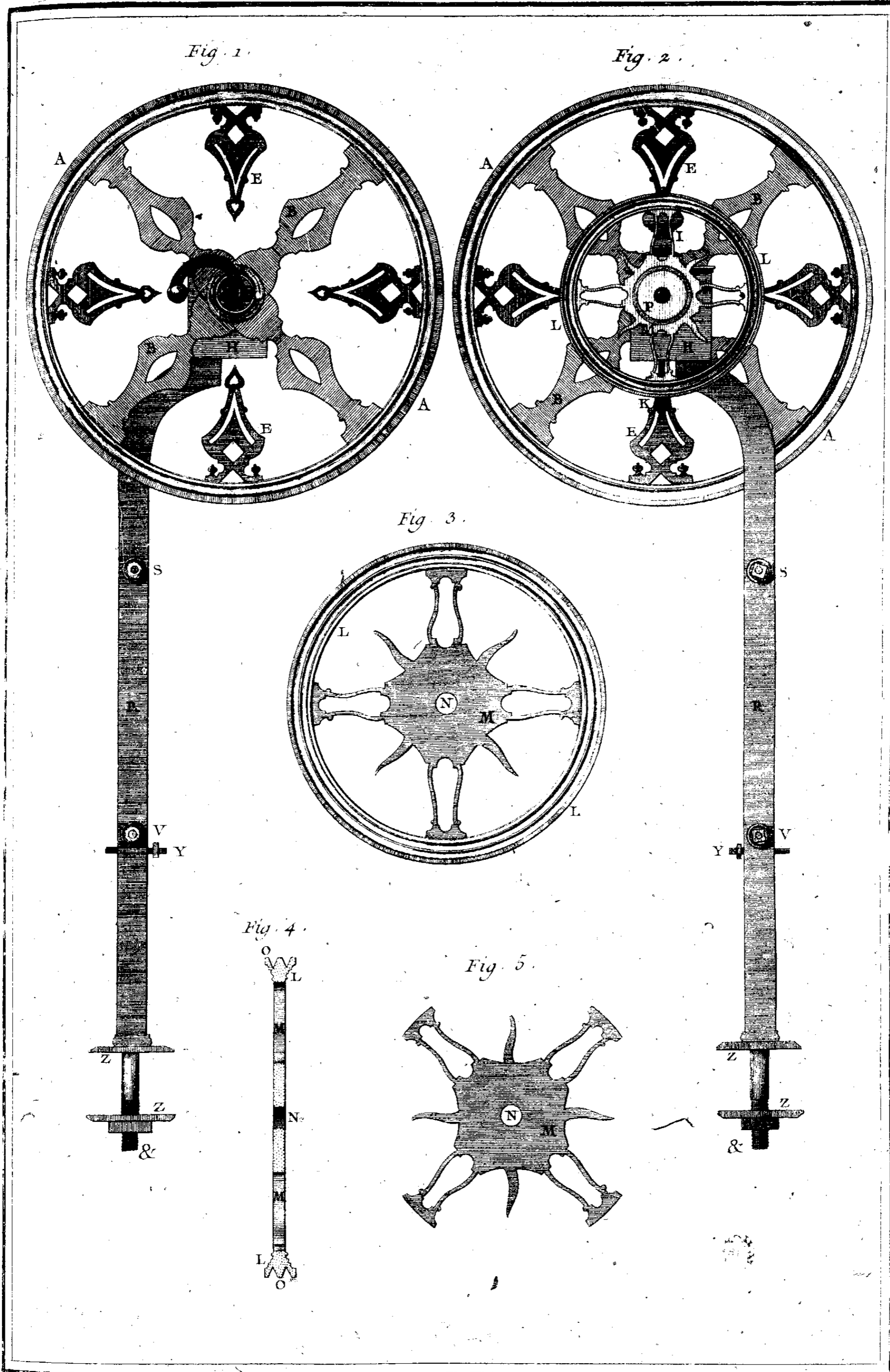
Tourneur, Tour à Figure; Face Laterale de la grande Roue et de son Support.
