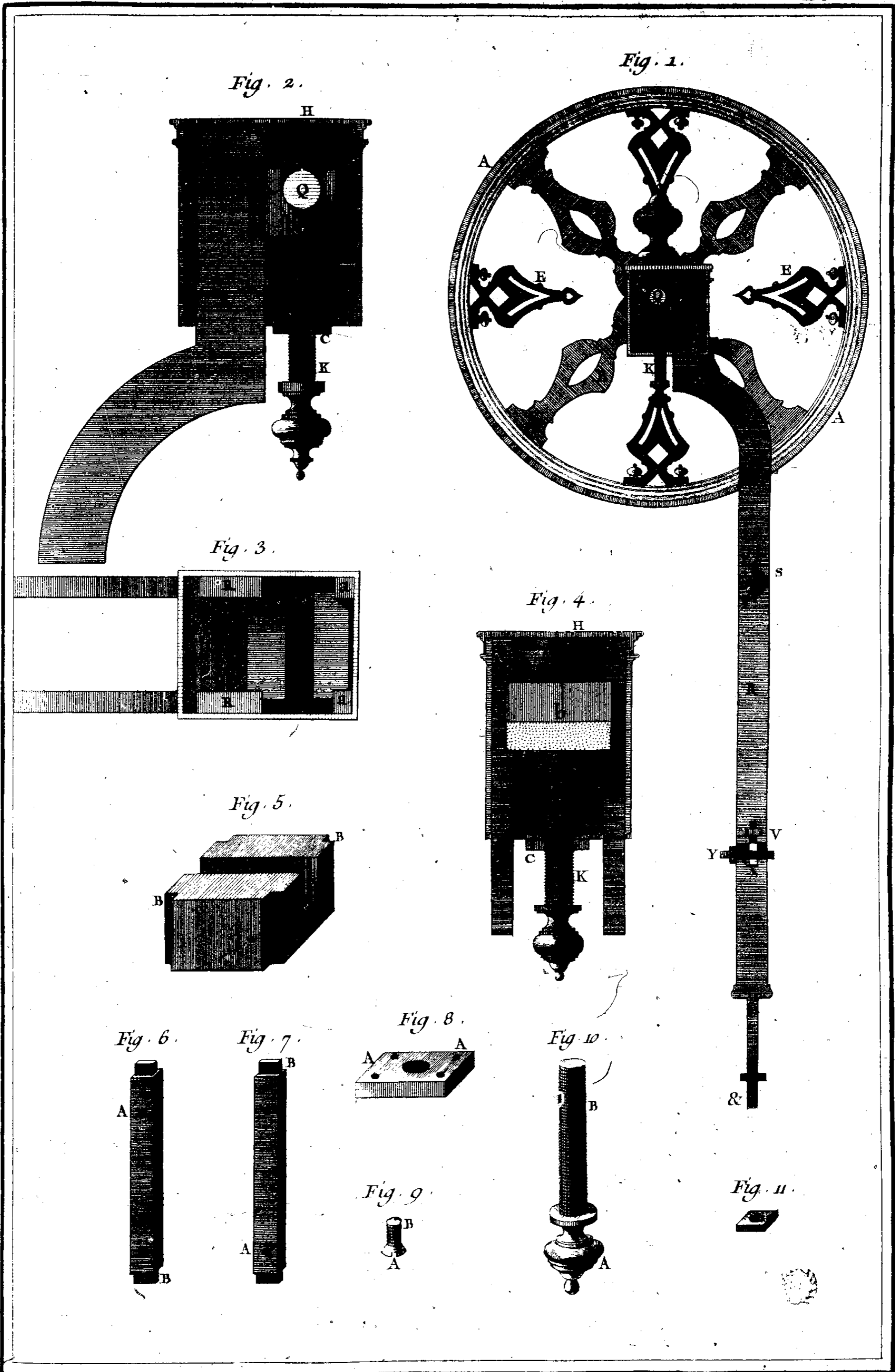
Tourneur, Tour à Figure, Coupe Latérale de la grande Roue et Détails.
