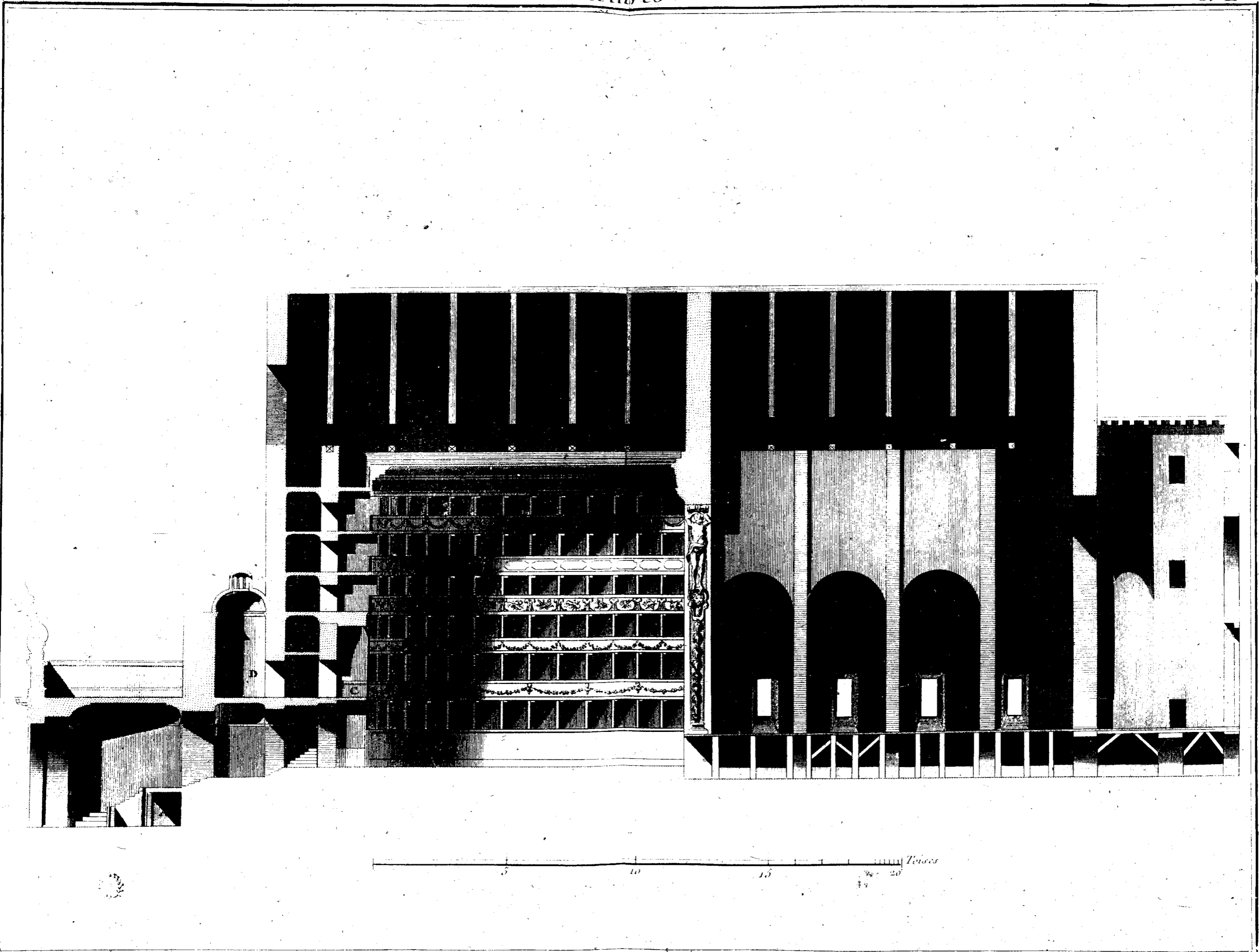
Salles de Spectacles, coupe du Théâtre Royal de St. Charles à Naples.
