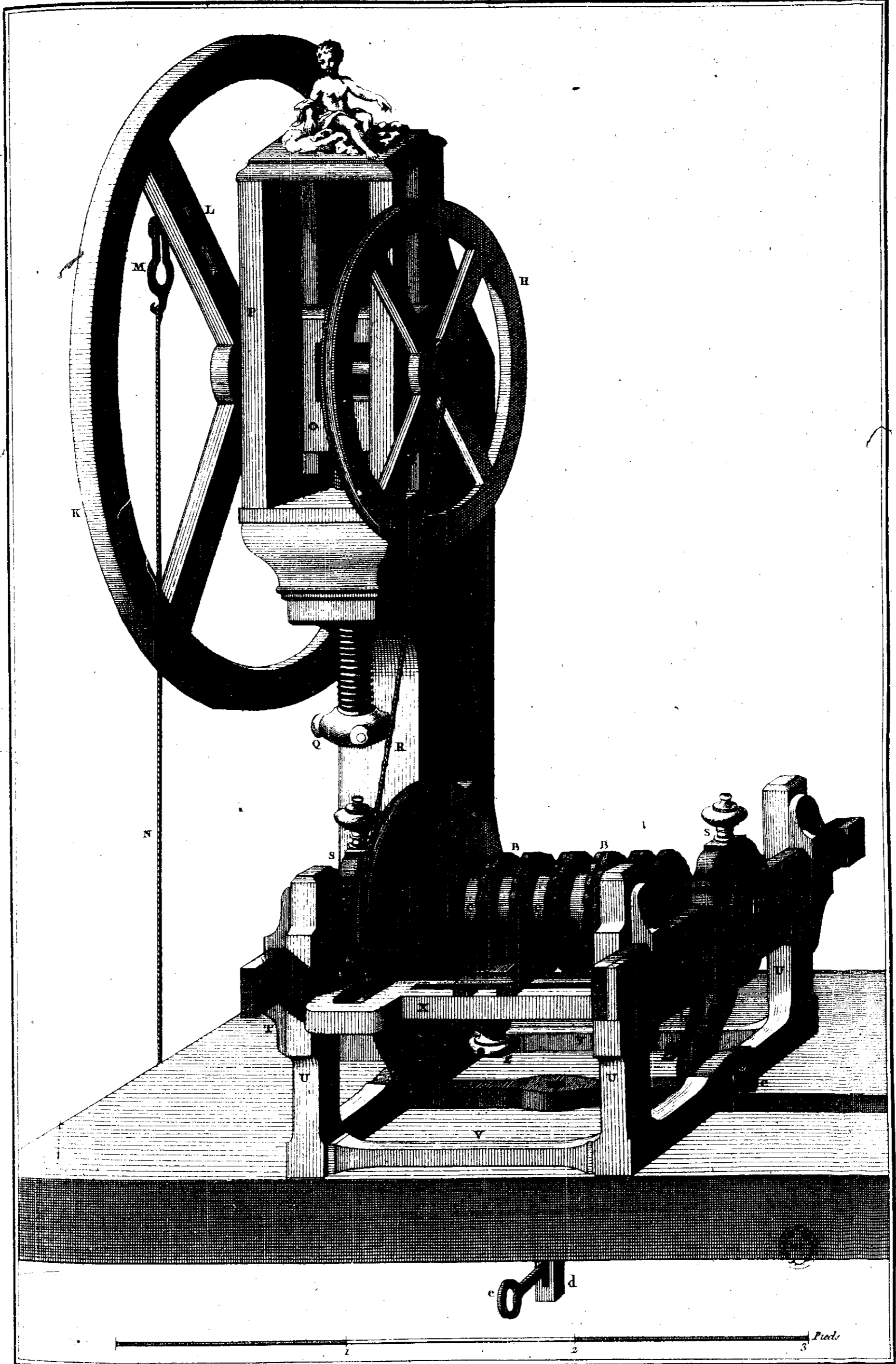
Tourneur, Tour à Guillocher à Roue
