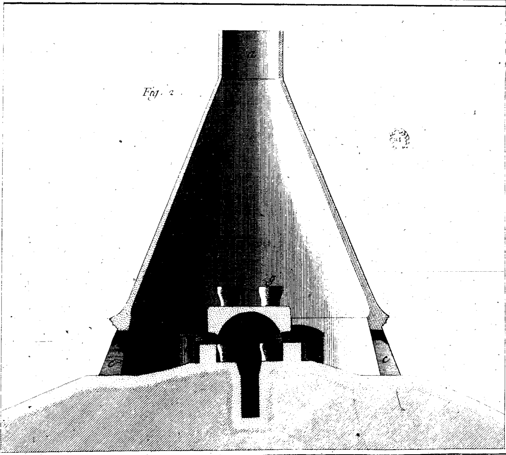
Verrerie Anglaise. Vue extérieure de la Verrerie, et Coupe sur la largeur.
