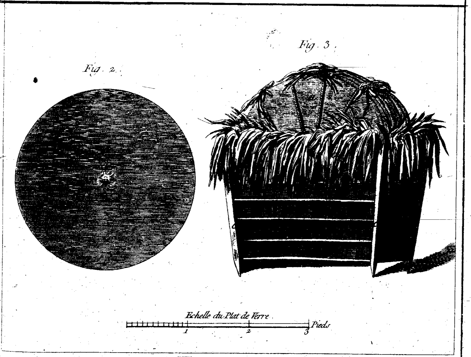
Verrerie en bois, Grande Verrerie à Vitres, ou en Plats. Extérieur d'une Halle, et Plat de Verre emballé.
