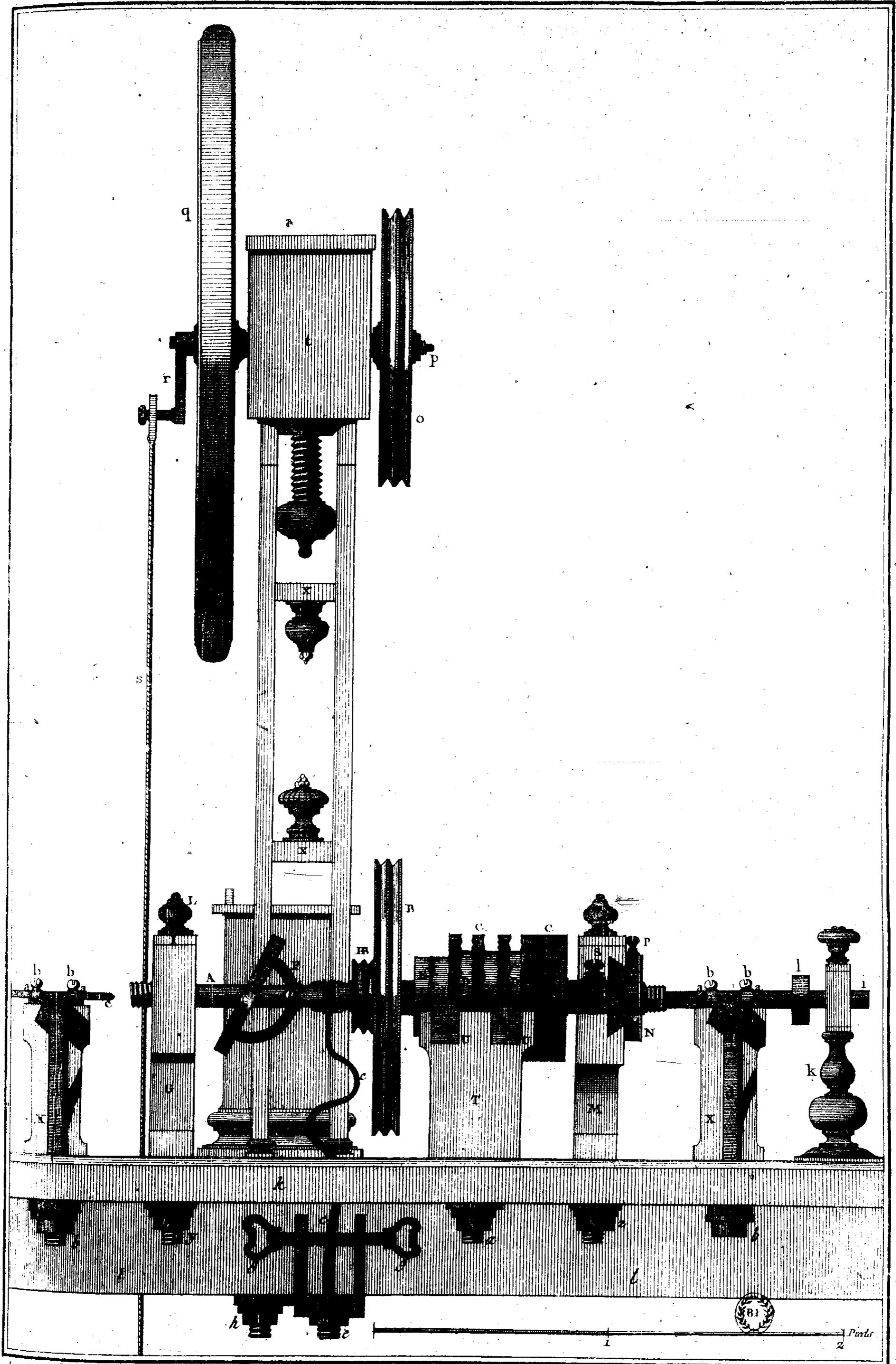
Tourneur, Tour a Guillochis avec Outils mobiles.
