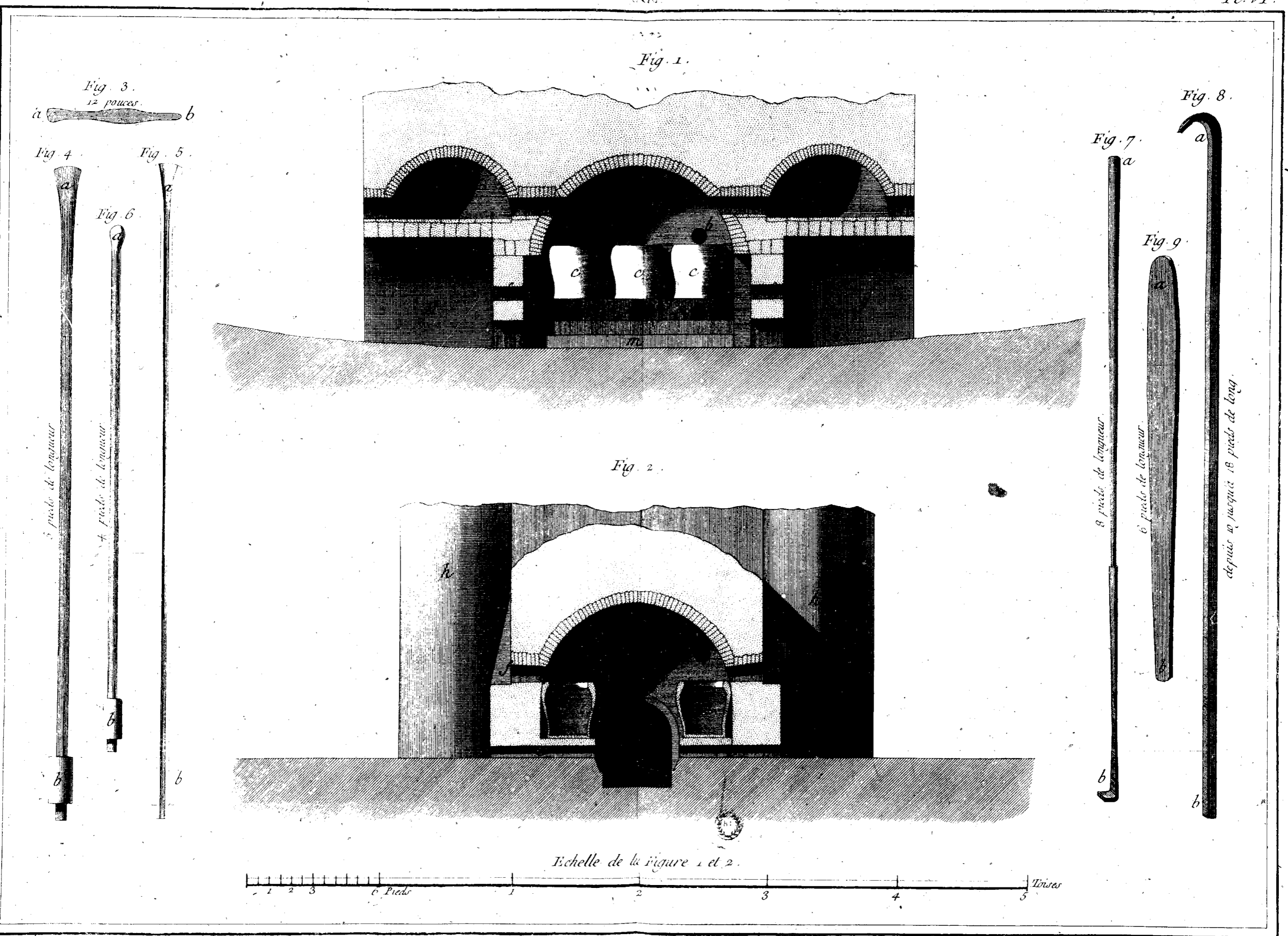
Verrerie en bois, coupes sur la longueur et sur la largeur d'un Four de grande Verrerie en Plats, et 5 differens Outils.
