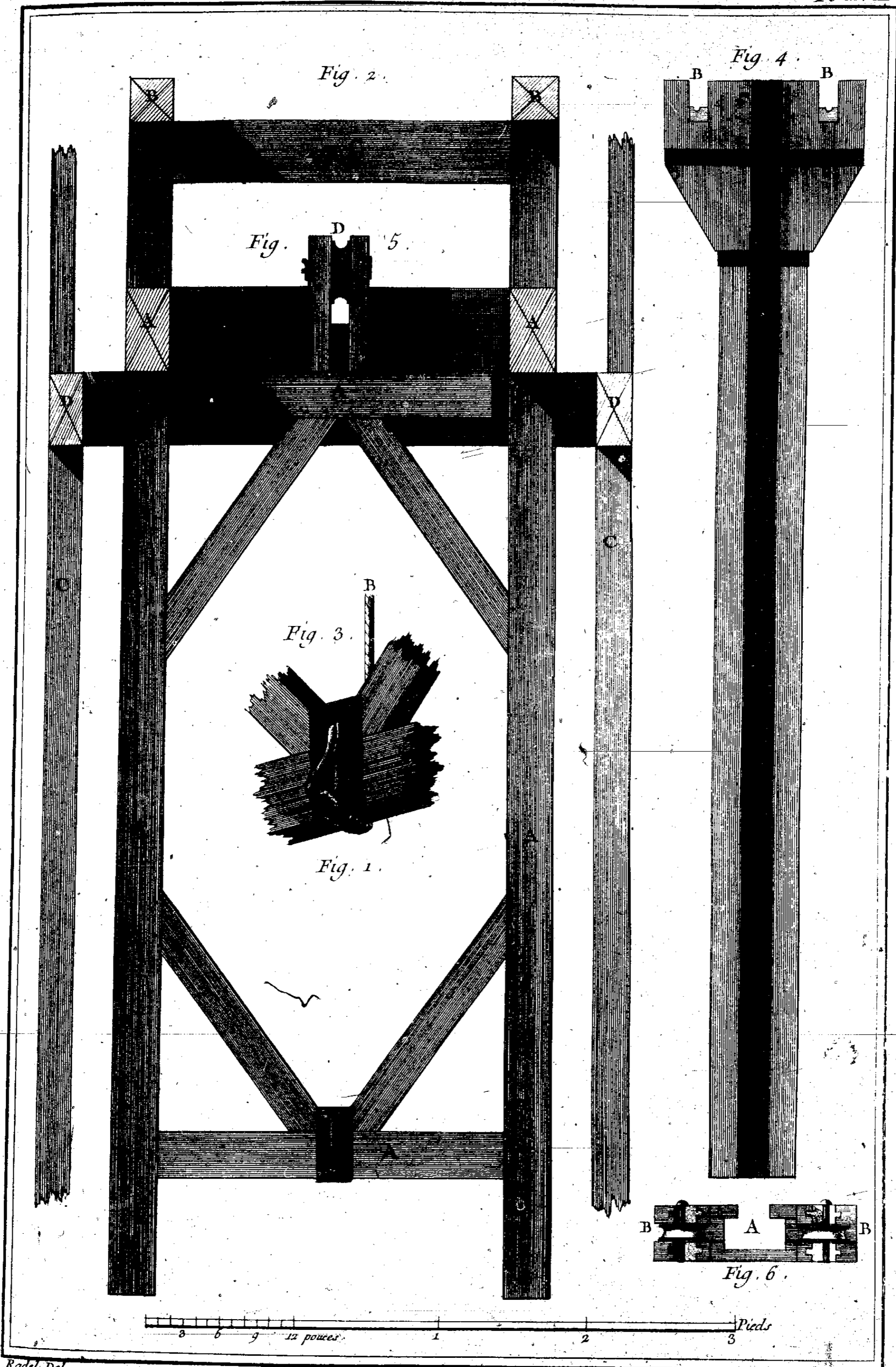
Machines de Théâtres, Elevation Géométrale des Batis servant d'une pour monter les Chemins centrés avec leurs Equipages R
