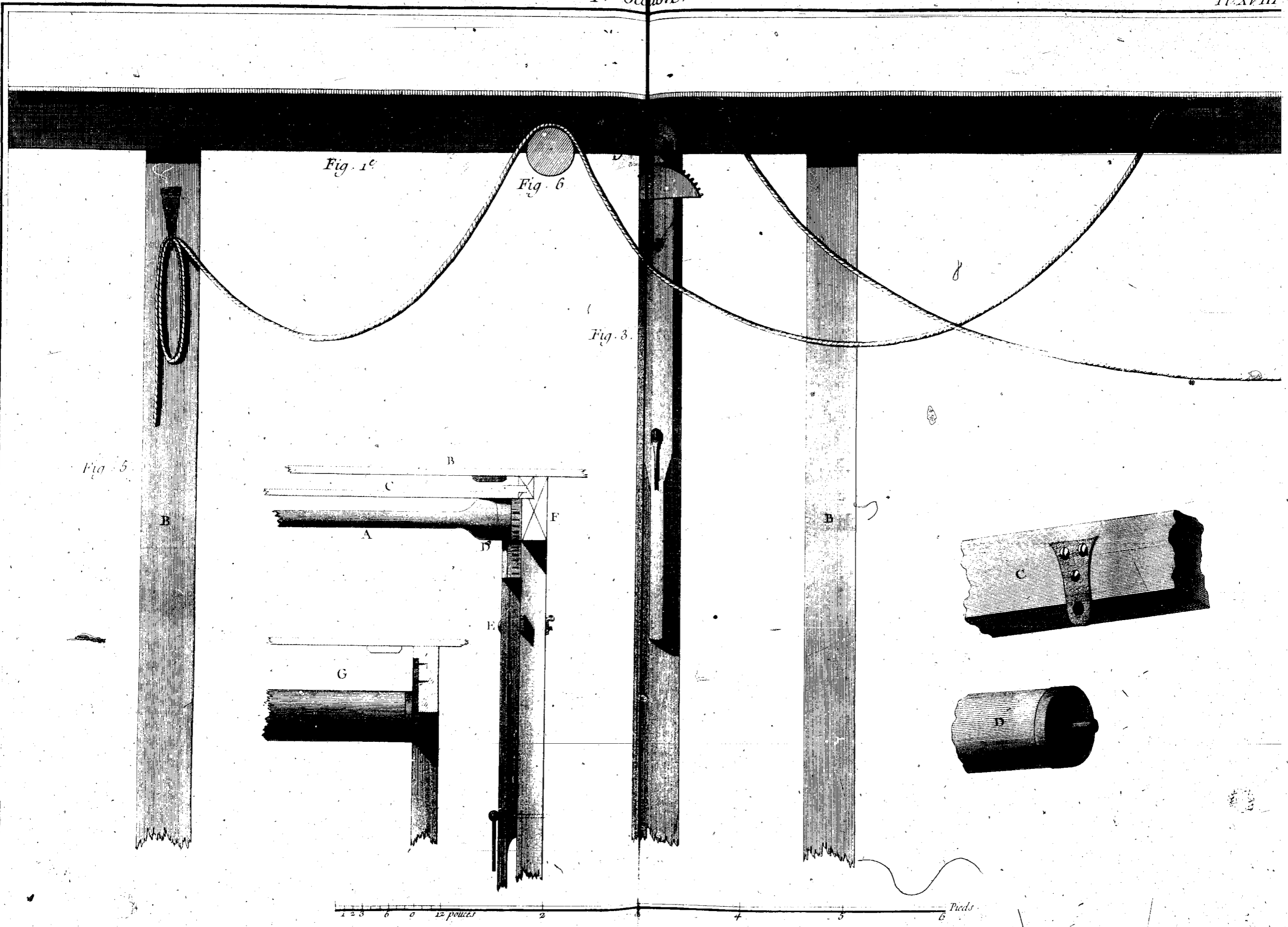
Machines de Théâtres, Coupe et Elevation sur la face de la Levée des Trapes avec la manivelle des Leviers et Engrainages des Rouleaux pour l'échappement des Trapes des grandes Rues, avec les Rouleaux sur lesquels passent les Trapes pour les ouvrir au besoin
