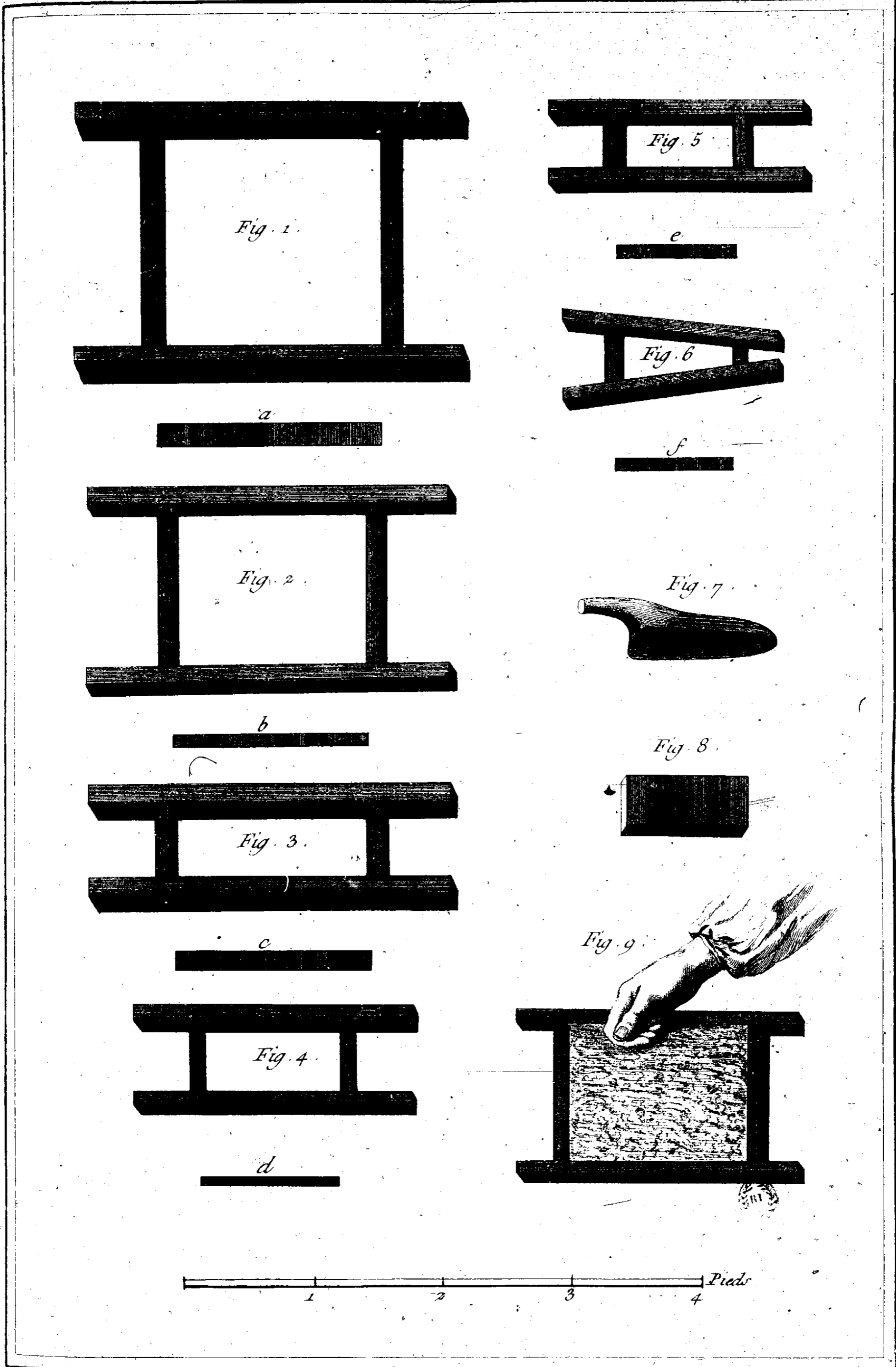
Verrerie en bois, Moules et proportions des Briques pour la construction du Four.
