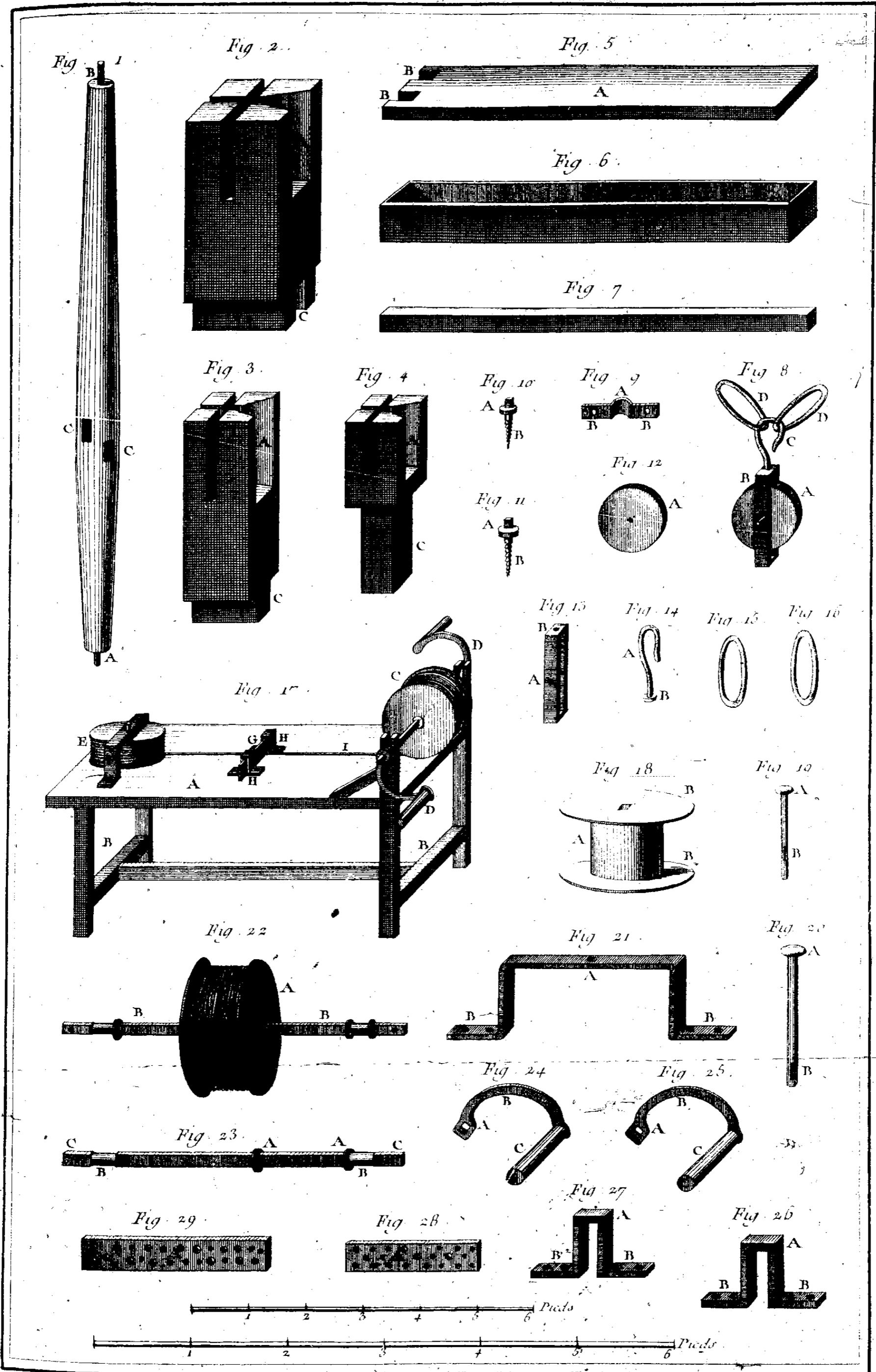
Fileur d'Or, Détails de l'Arguc et Moulins à tirer la Gavette
