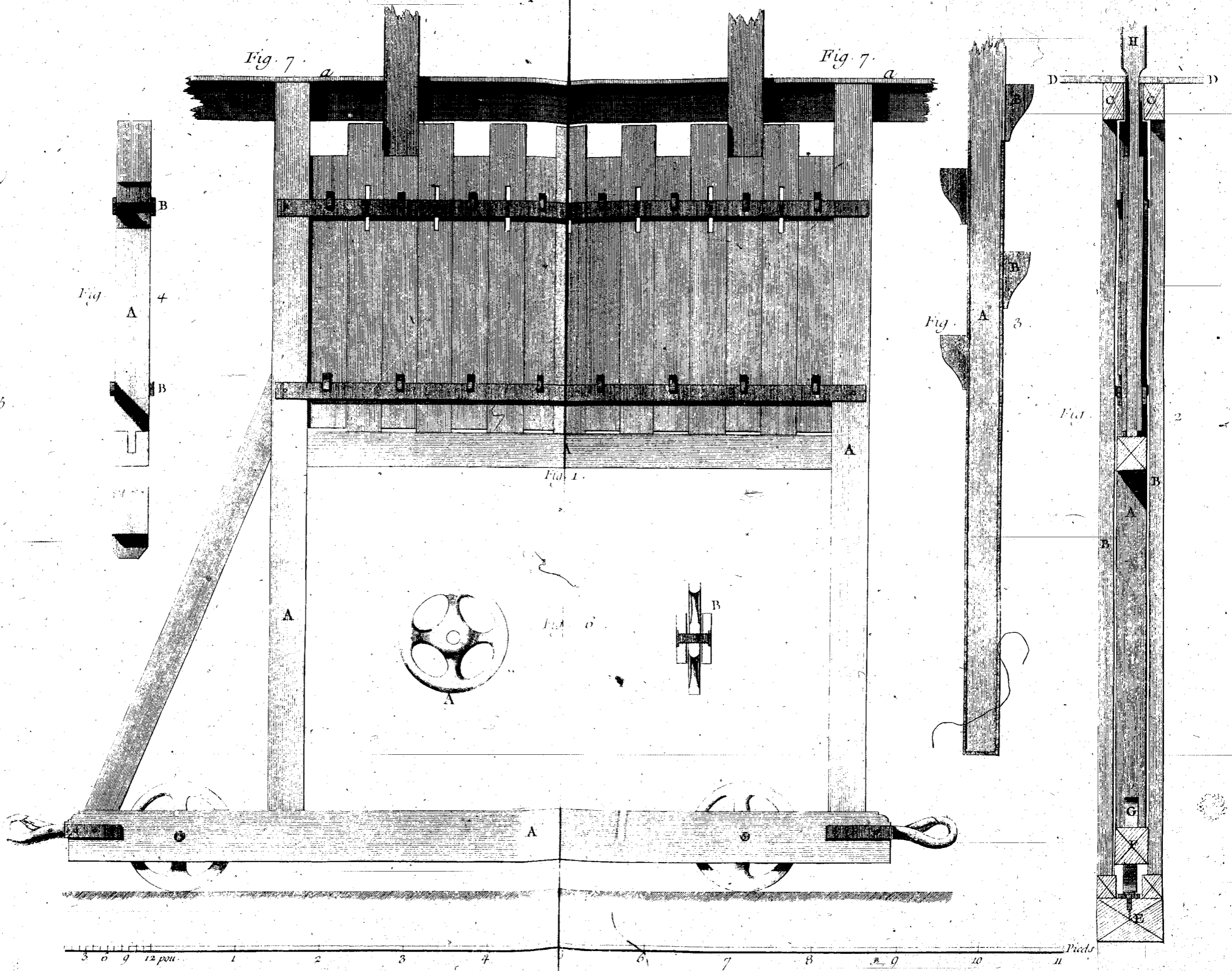
Machines de Théâtres, Chariot du 8 au 13 pour le service des Décorations Pittoresques détaillées dans la Planche quatorze
