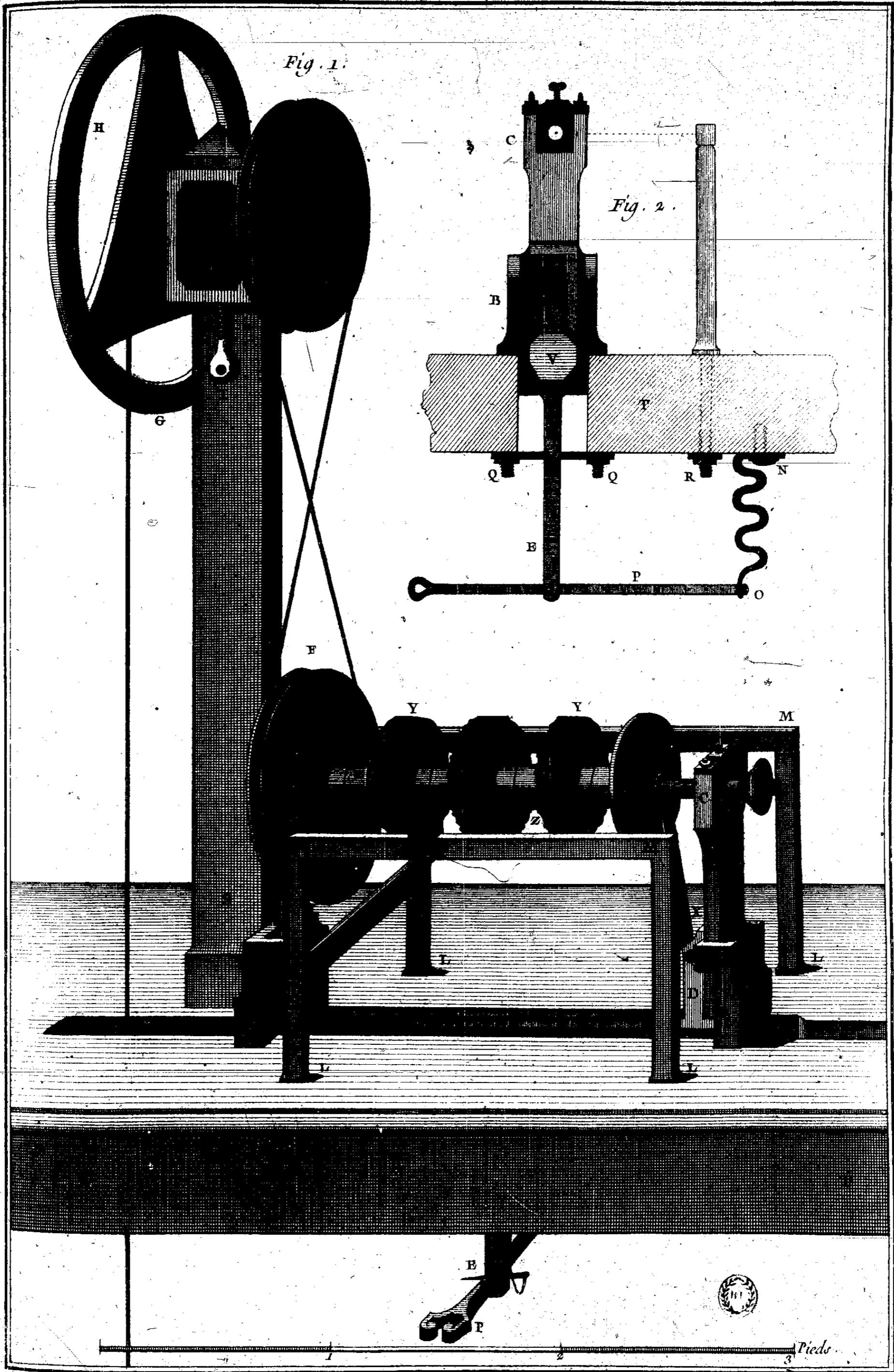
Tourneur, Tour à Guillocher à Roue.
