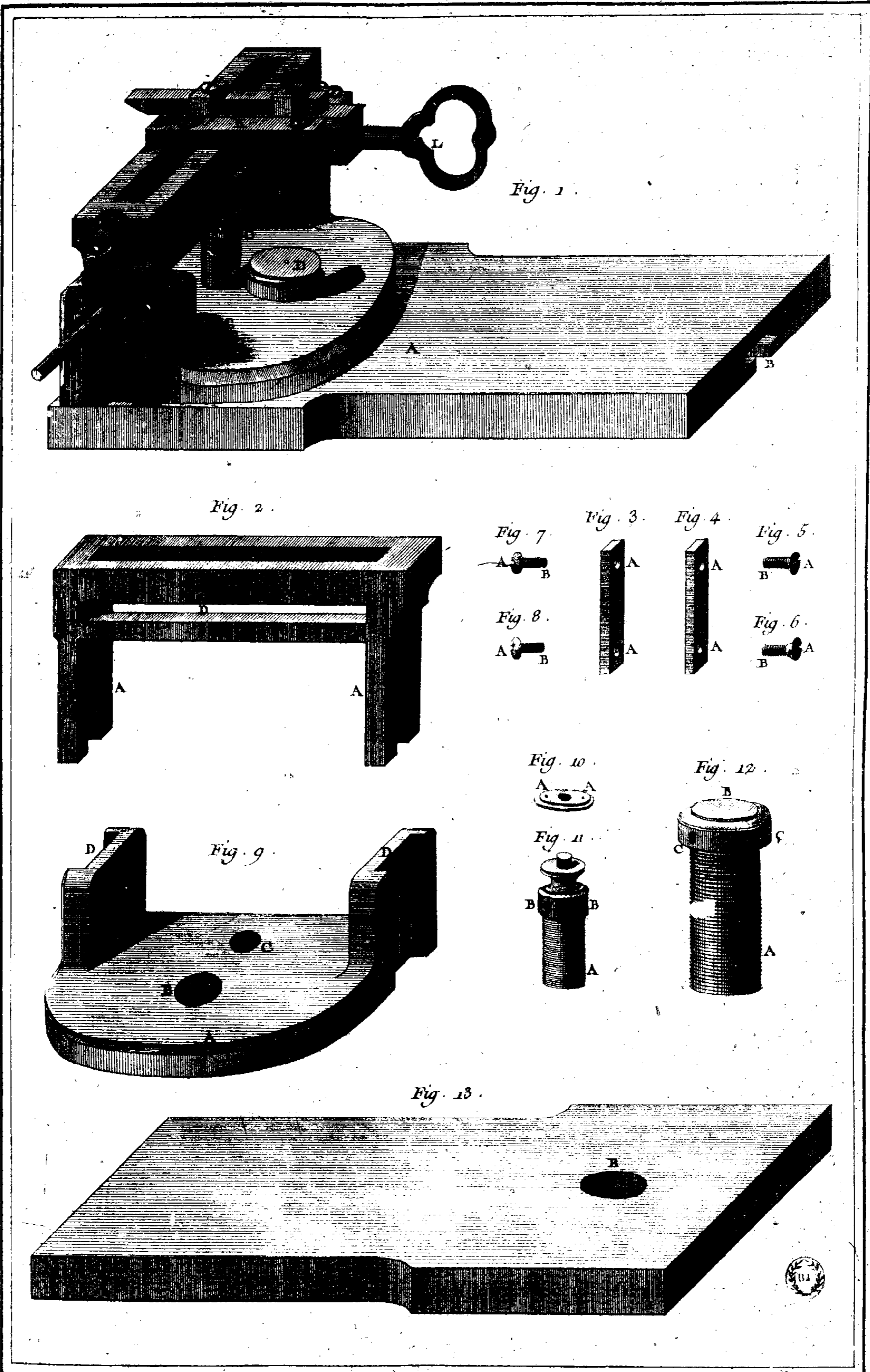
Tourneur, Tour à Figure; Support à pivot et Détails.
