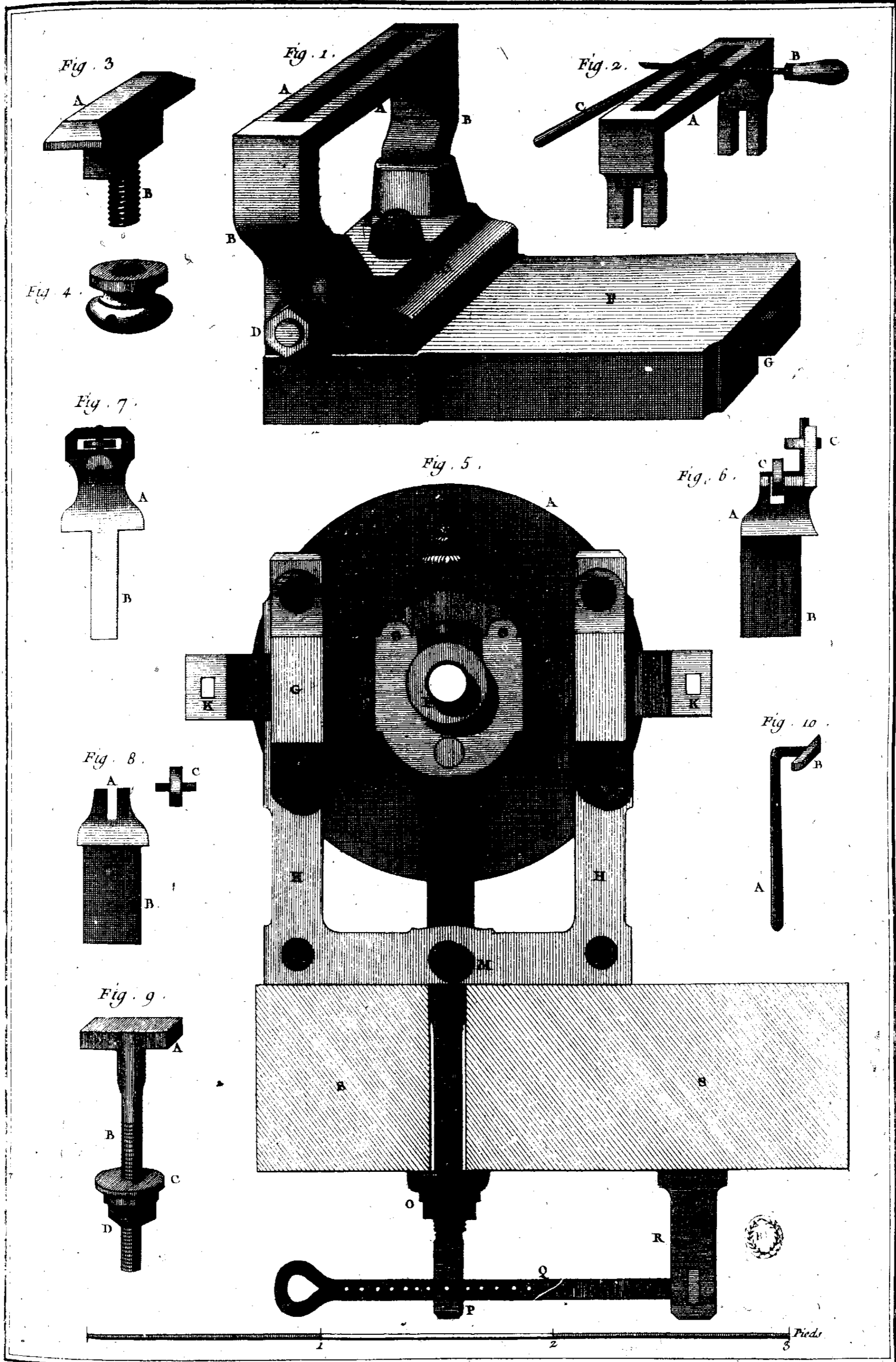
Tourneur, Détails du Tour à Guillocher à Roue ?
