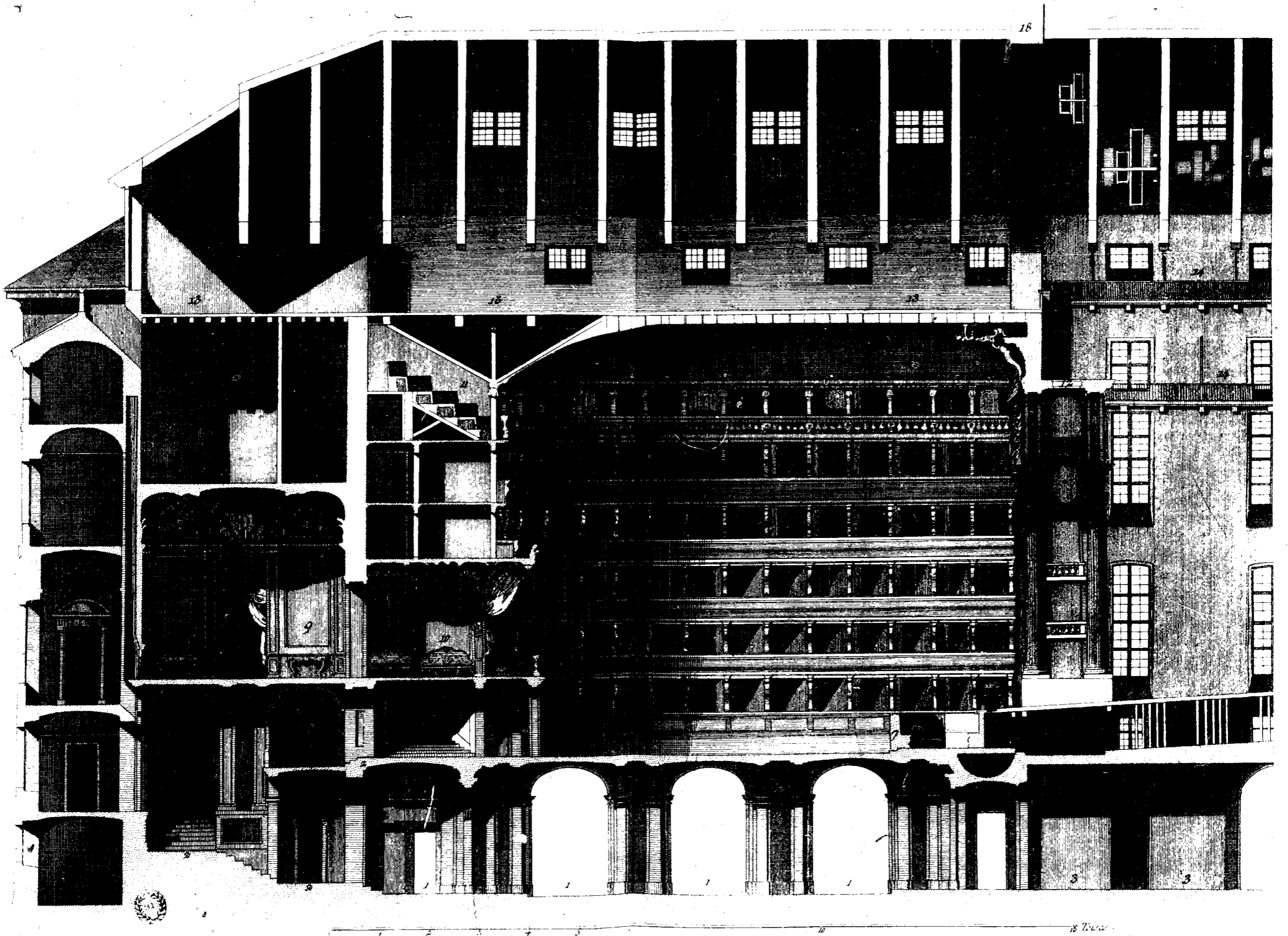
Salles de Spectacles coupées sur toute la longueur du Théâtre de Turin.
