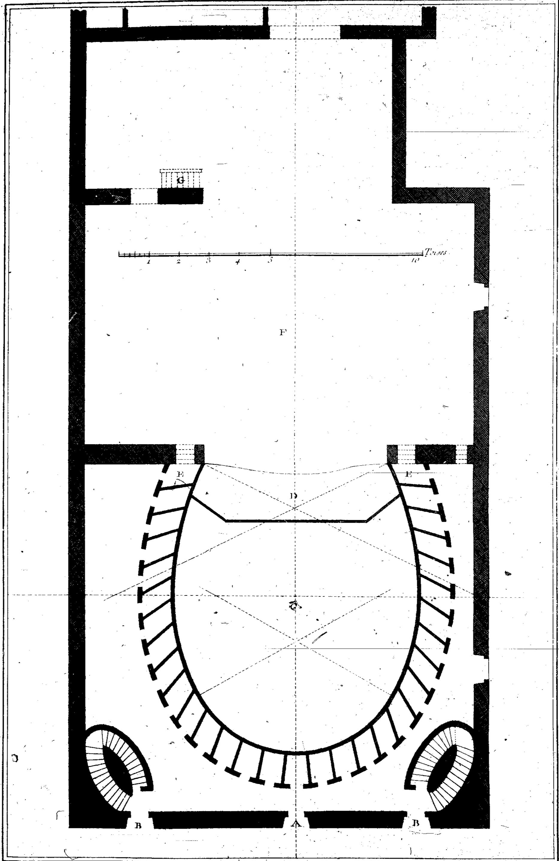
Salles de Spectacles Plan du Théâtre d'Argiletum à Rome
