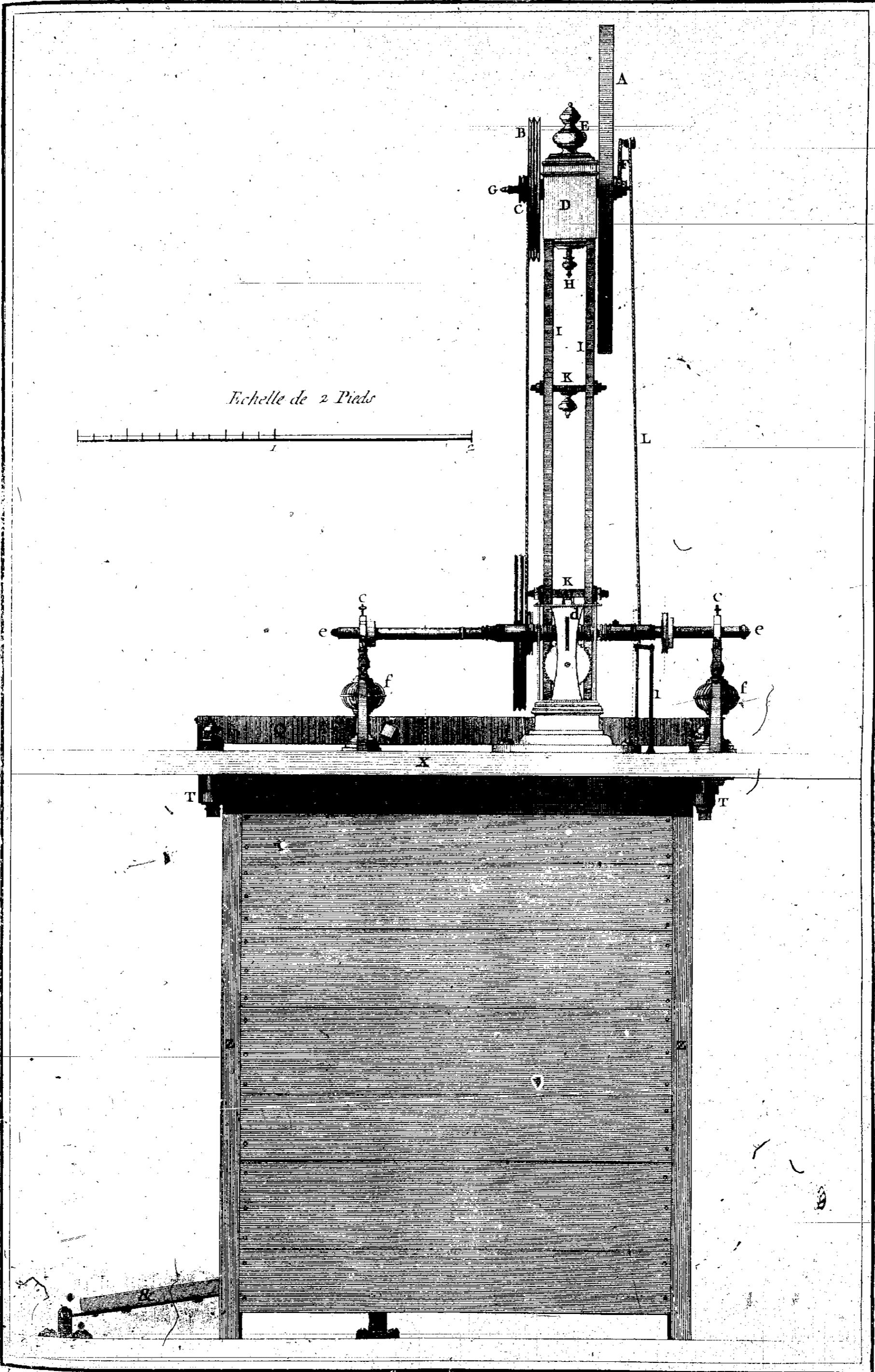
Tourneur, Tour à Figure, Elevation par derriere.
