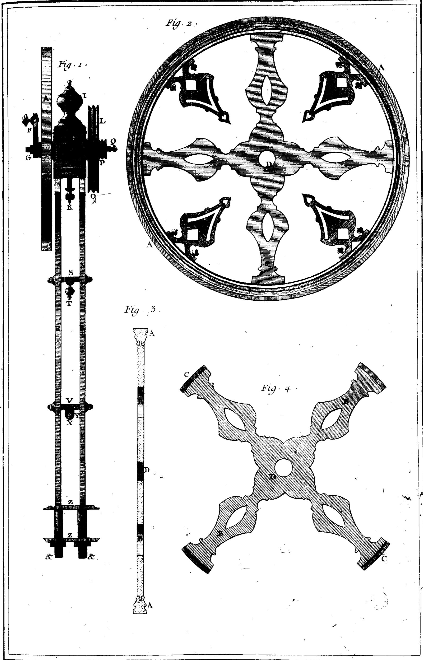
Tourneur, Tour à Figure, vue en face de la grande Roue.
