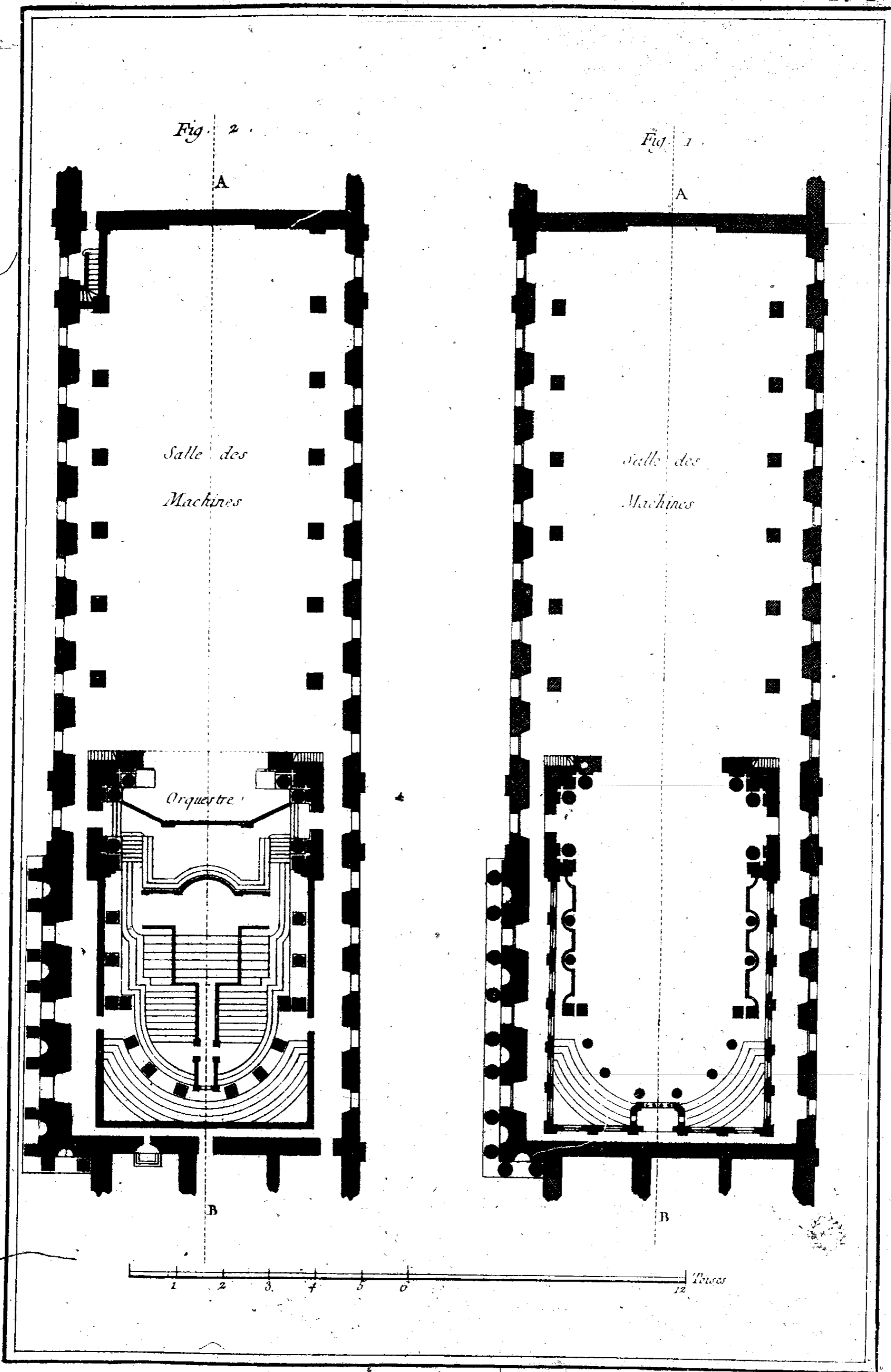
Salles de Spectacles, Plan au Rez de Chaussée, et Plan a la hauteur des premieres Loges de la Salle des Machines du Château des Thuilleries
