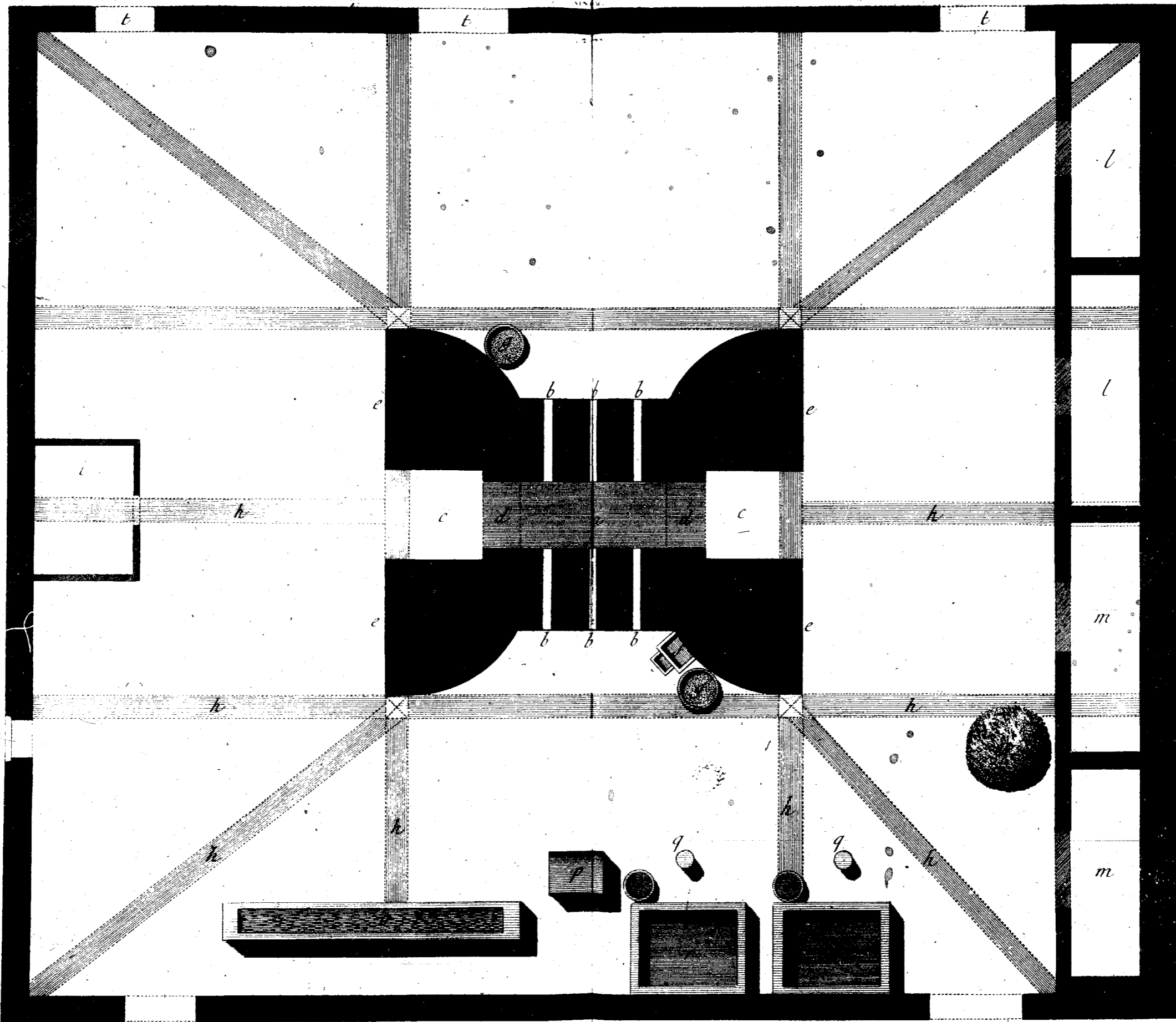
Verrerie en bois, Plan Général d'une grande Verrerie en Plats.
