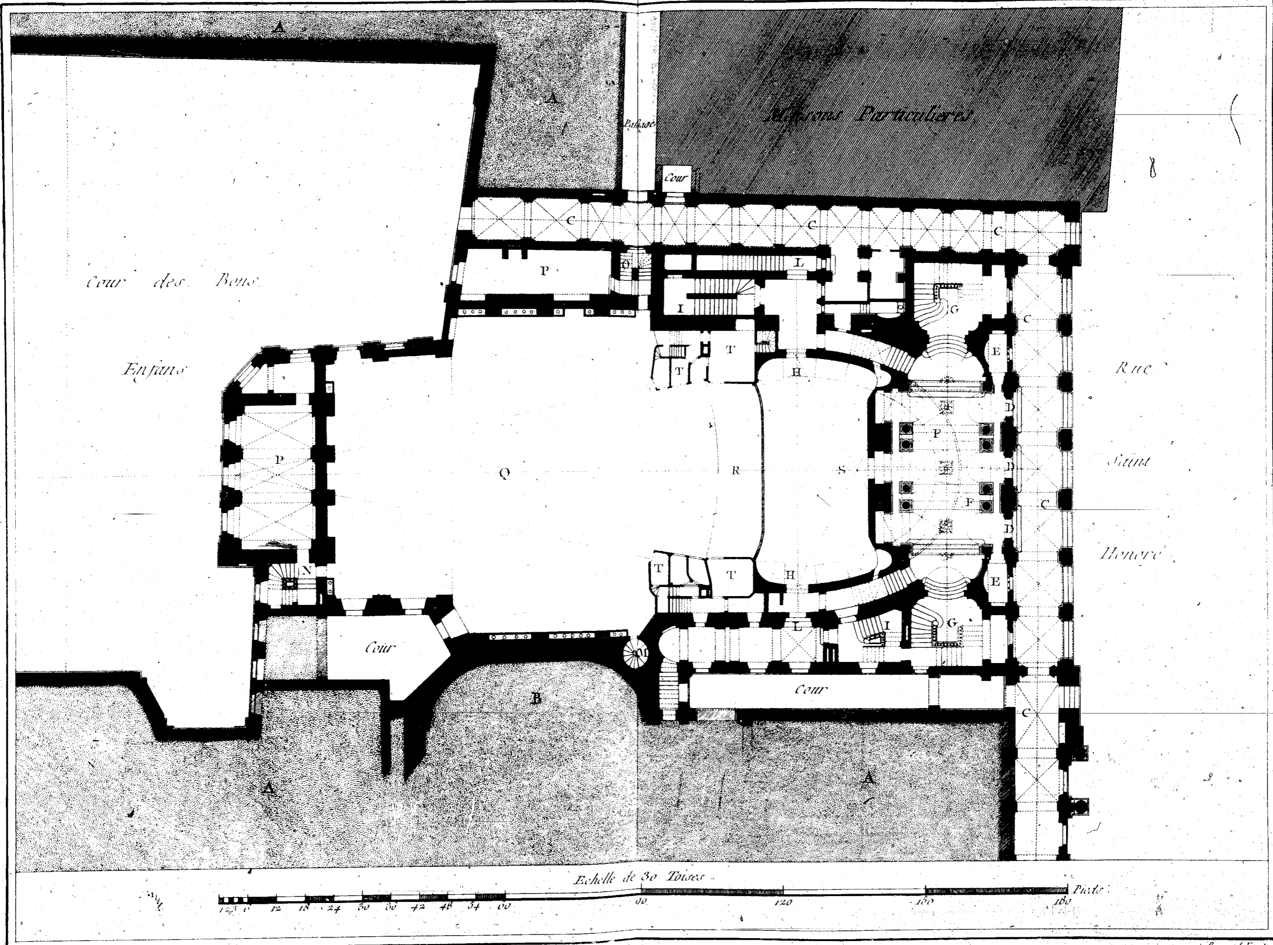
Salles de Spectacles, Plan au Rez de Chaussée du Parterre de la Nouvelle Salle de l'Opera, Exécutede au Palais Royal sur les Dessains de M. Moreau Architecte du Roy et de la Ville
