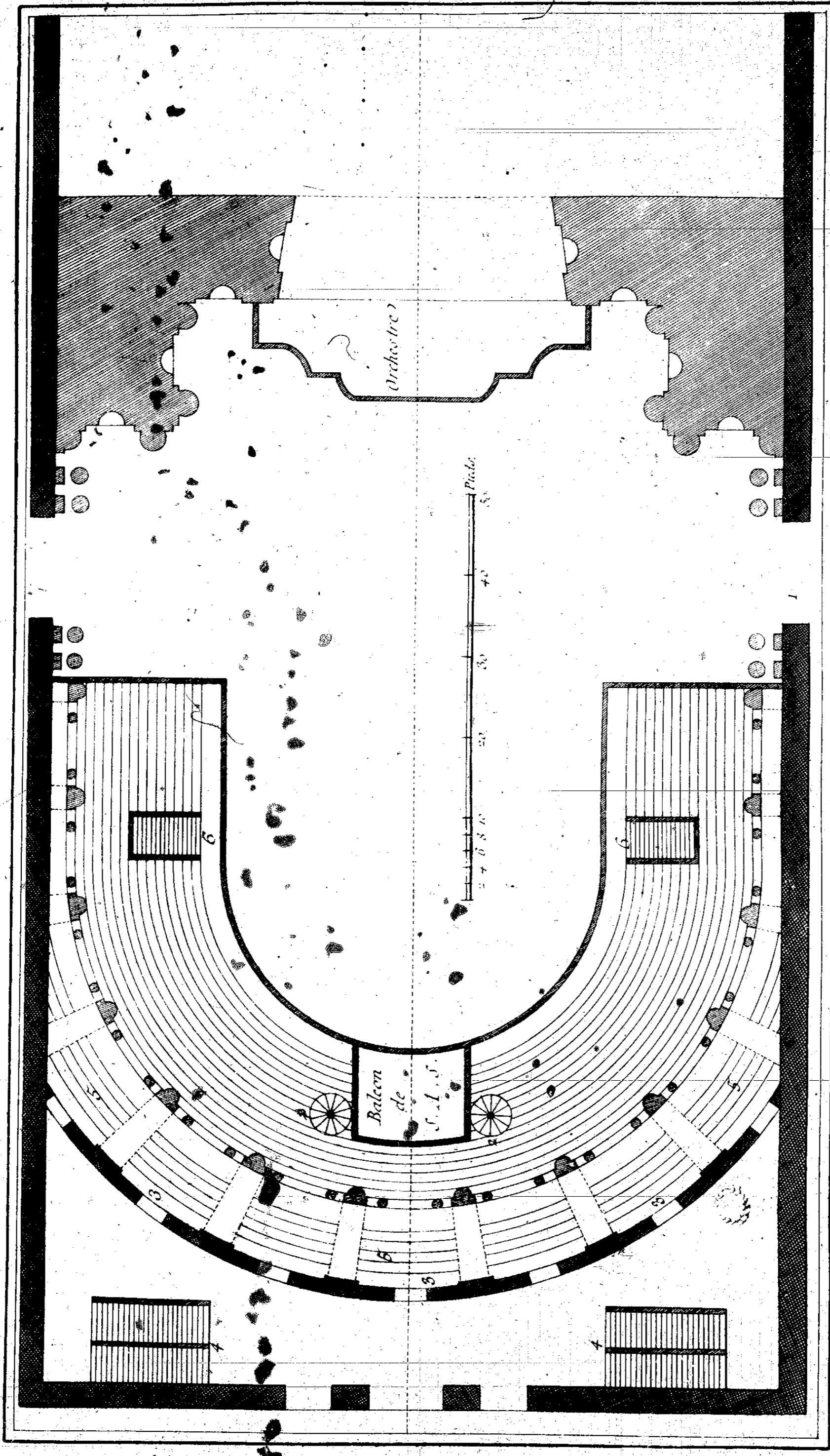
Salles de Spectacles, Plan du Theatre de Parme
