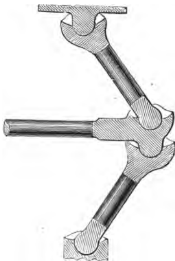
Fig. 39.—Knuckle-joint.
