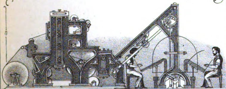
WALTER PRESS
