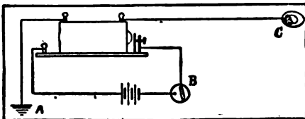
Shocking-Machine
