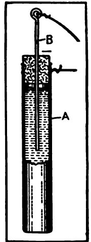
Water Rheostat
