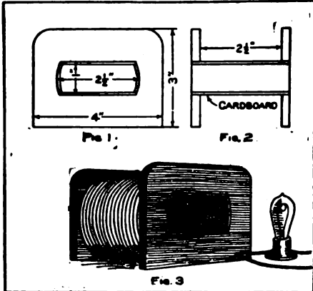
Watch Demagnetizer
